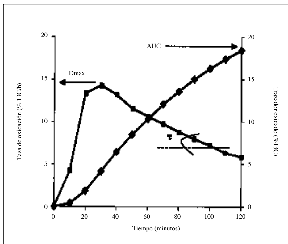
Fig. 1.—Parámetros que describen el proceso de oxidación obtenidos a partir del test en aliento con 2-ceto[1- 13 C]isocaproato: porcentaje de trazador oxidado o área bajo la curva de oxidación (AUC), tasa máxima de oxidación ( D_{\text{max}} ) y constante de velocidad ( \tau ).
