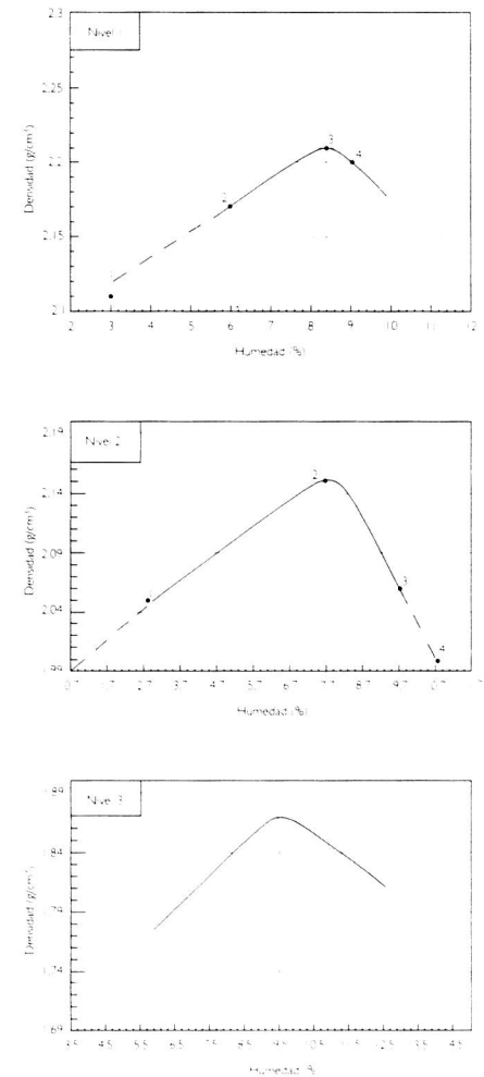
Figura 6 Curvas de compactación óptima
