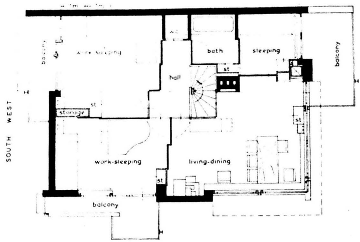
3. Casa Schroeder. Planta alta.
