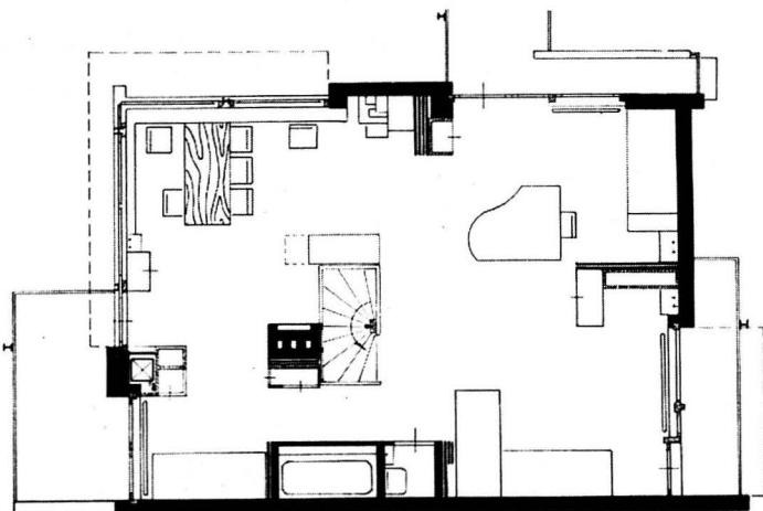
4. Casa Schroeder. Planta alta.
