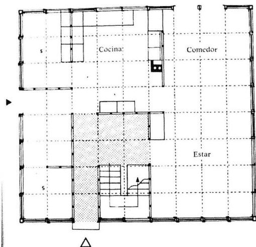
6. Gropius: Vivienda prefabricada en la colonia Weissenhof.
