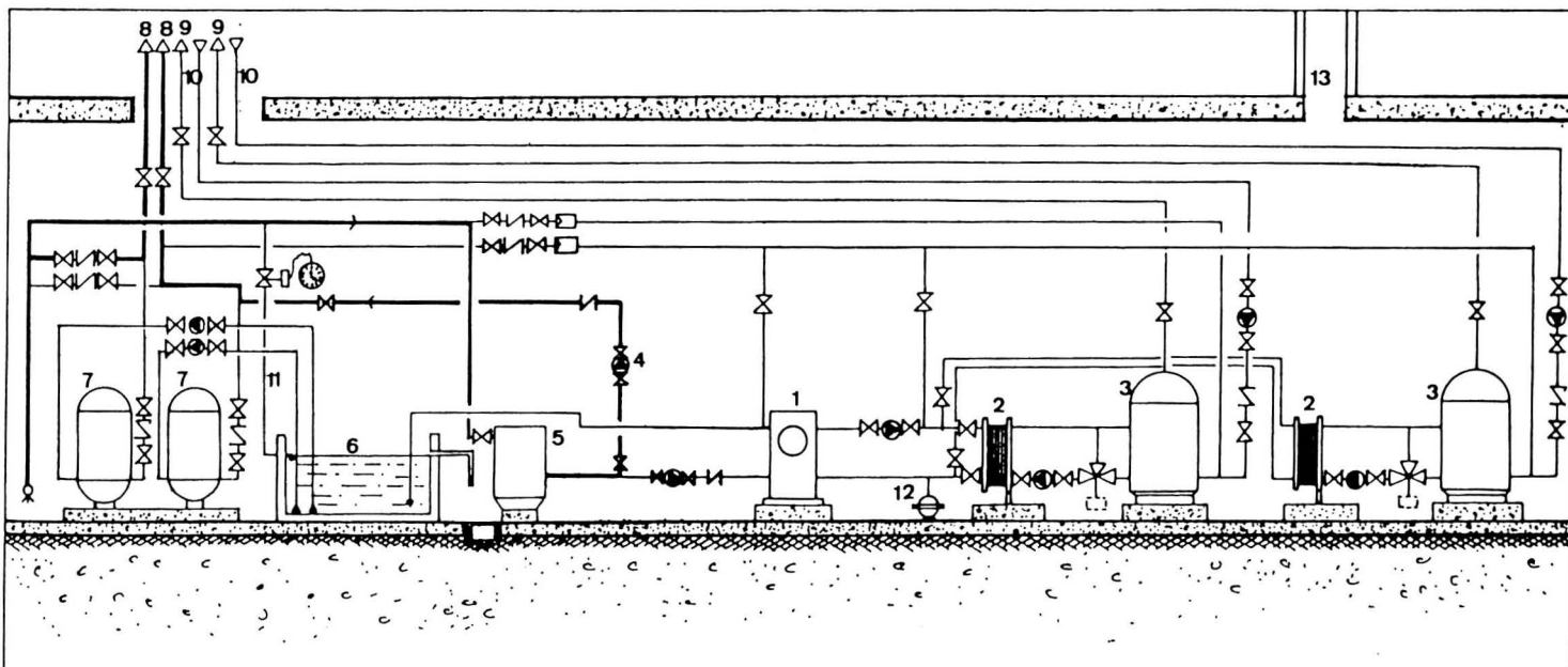
FIGURA 5. PREPARACION DE ACS CON AGUA DE ABASTECIMIENTO COMO FUENTE ENERGETICA
