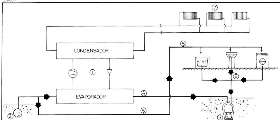
FIGURA 2. AGUA DE ABASTECIMIENTO COMO FUENTE ENERGÉTICA: DISEÑO INADECUADO
