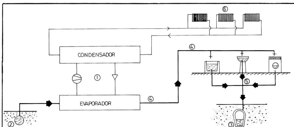
FIGURA 3. AGUA DE ABASTECIMIENTO COMO FUENTE ENERGÉTICA: DISEÑO IDÓNEO
