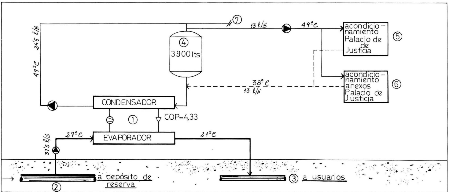
FIGURA 6. ACONDICIONAMIENTO TERMICO DE LOCALES CON AGUA DE ABASTECIMIENTO COMO FUENTE ENERGETICA
