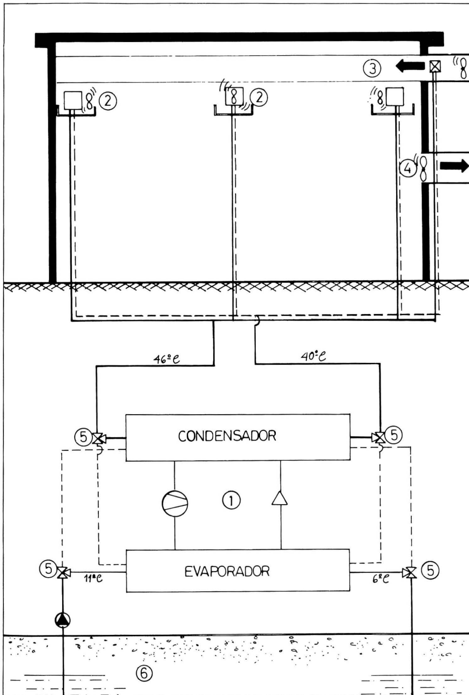
FIGURA 1. BOMBA DE CALOR AGUA-AGUA CONVENCIONAL
