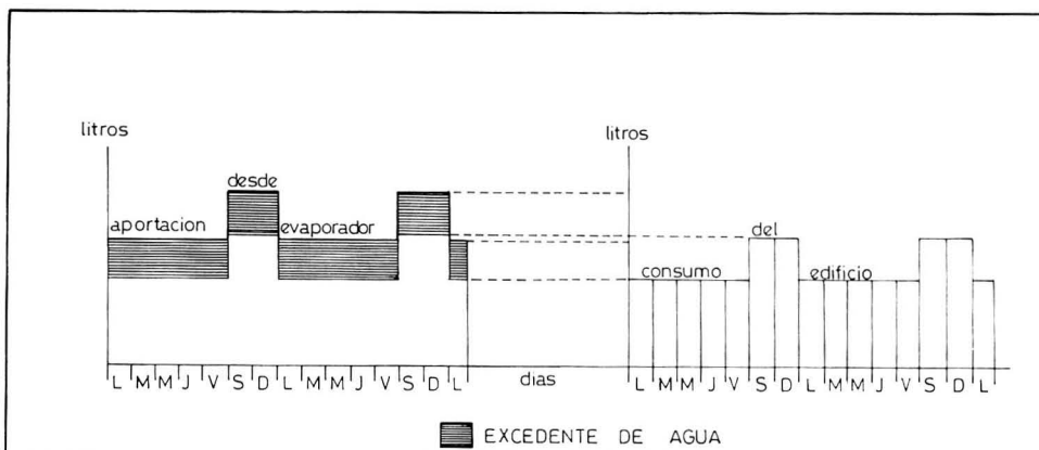
FIGURA 4. PERFILES DE CONSUMO Y APORTACIONES DE AGUA DESDE EL EVAPORADOR
