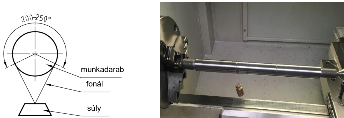
4. ábra. Fonálmódszer elvi a) és gyakorlati b) elrendezése [9]
