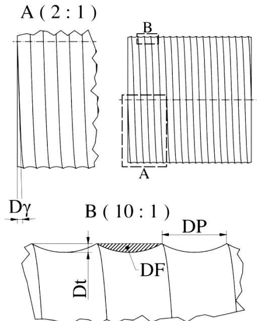
1. ábra. Sodratos felület paramétereit [5]
