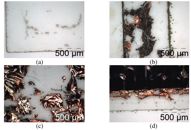
Fig. 3. Printed pattern after sintering (a) 2200 V, 1700 \mu\text{s} (b) 2000 V, 1500 \mu\text{s} (c) 2000 V, 1300 \mu\text{s} (d) 1800 V, 1000 \mu\text{s} .
