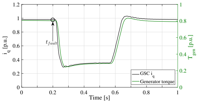
(d) Generator torque and i_q current of GSC
