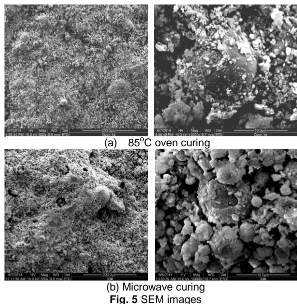
Fig. 5 SEM images
