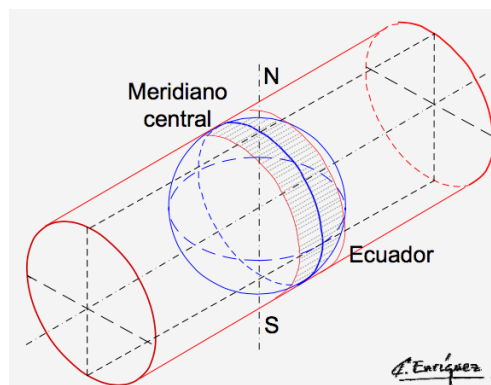
Ilustración 6. Modelo de Proyección UTM
