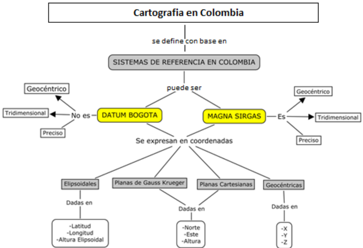
Ilustración 1. Sistemas de Referencia utilizados en Colombia Fuente: construcción propia.
