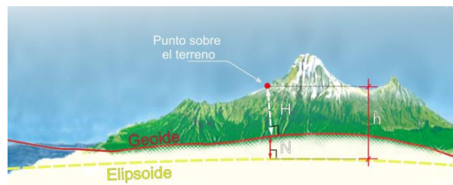
Ilustración 2. Esquema de Elipsoide. Fuente INEGI, 2004.
