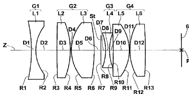
Рис. 1. Оптична схема об'єктива з патенту [11]
