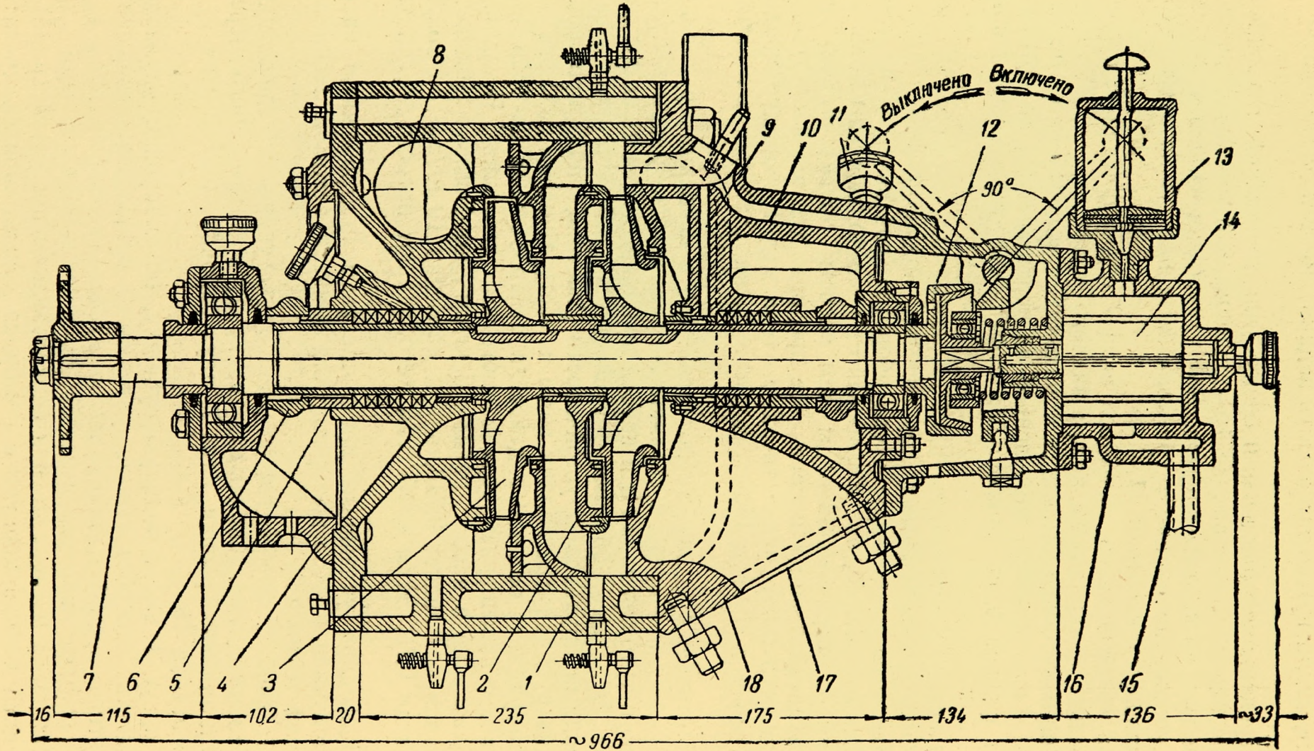
Фиг. 25. Разрез насоса центробежного типа.
