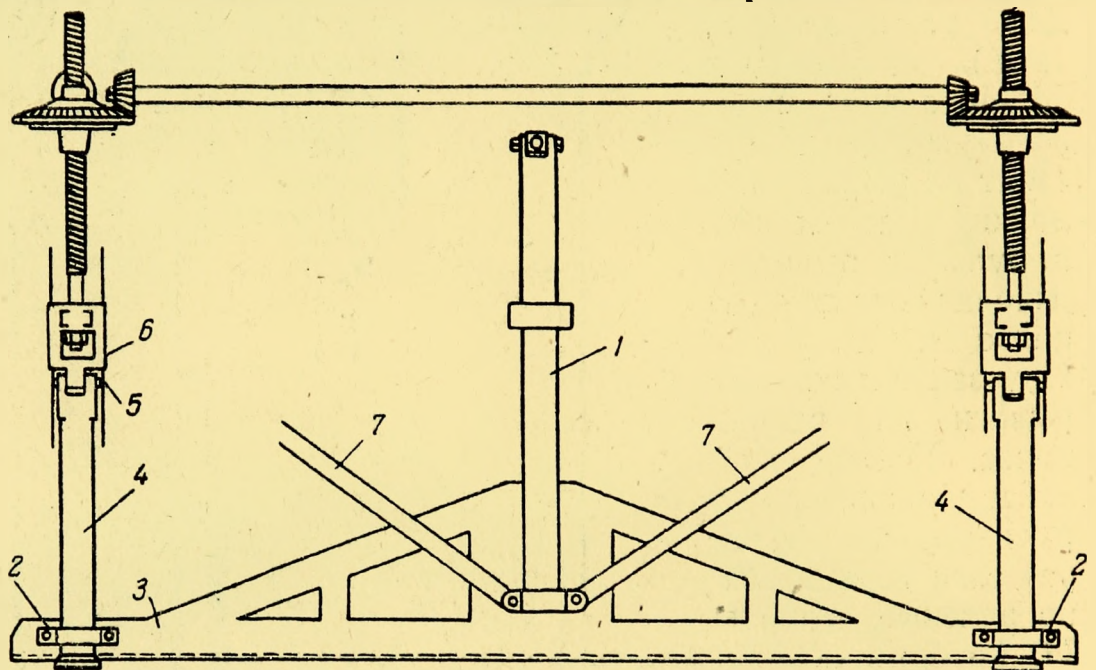
Фиг. 49. Схема подъемного механизма (вид сбоку).
