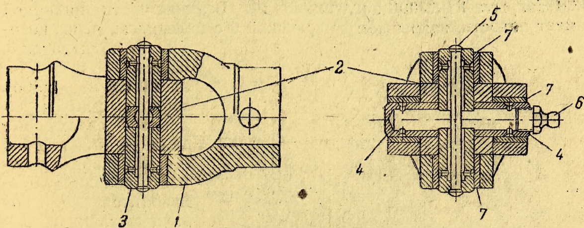
Фиг. 70. Карданное сочленение.
