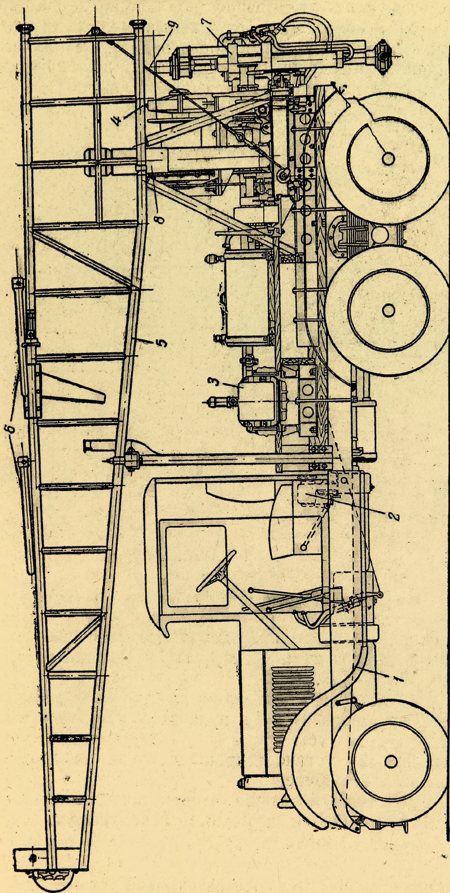
Фиг. 18. Автомобиль — буровая установка: 1 — шасси автомобиля; 2 — коробка отбора мощности; 3 — грязевой насос; 4 — лебедка; 5 — вышка; 6 — рабочие площадки; 7 — привод шпинделя; 8 — домкрат для опускания и постановки вышки; 9 — канат.
