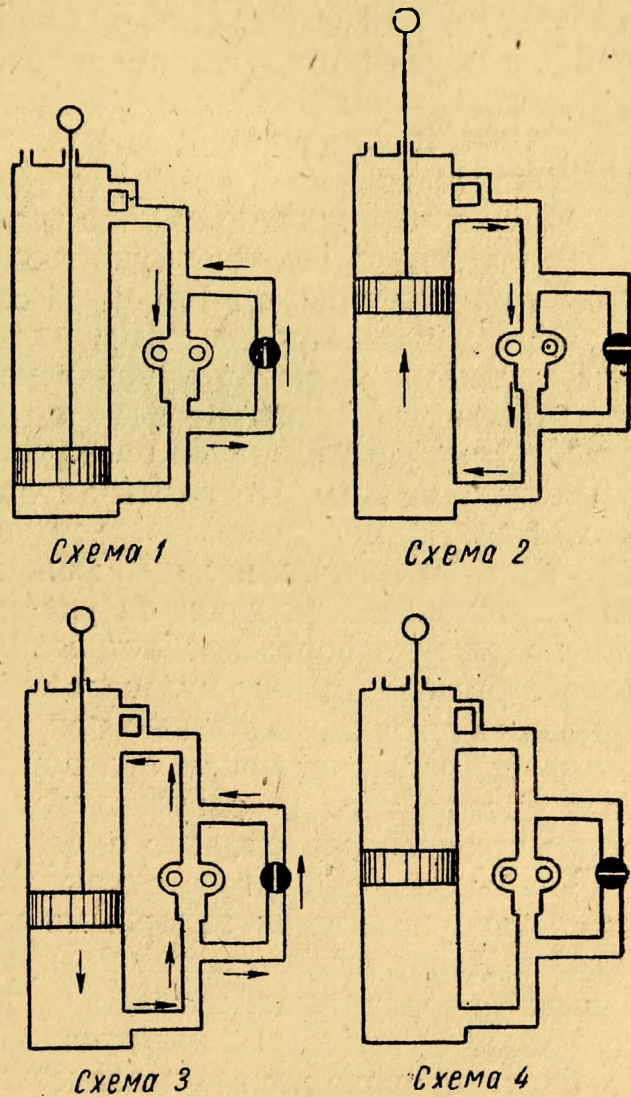
Фиг. 73. Схема работы гидроподъемника.
