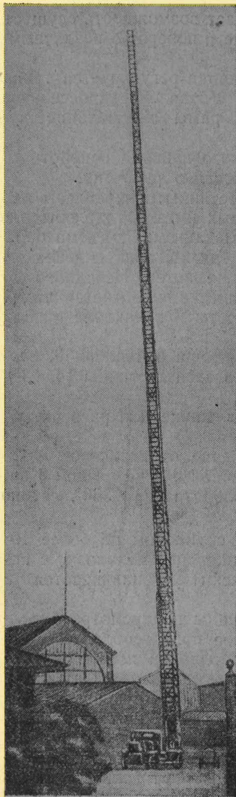
Фиг. 32. Автомеханическая лестница в развернутом виде.
