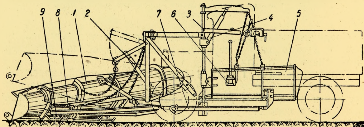
Фиг. 13. Схематический чертеж снегоочистителя Д-151.
