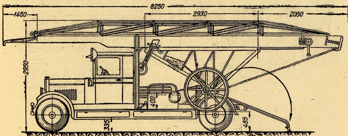
Фиг. 29. Автомобильная съемная лестница.
