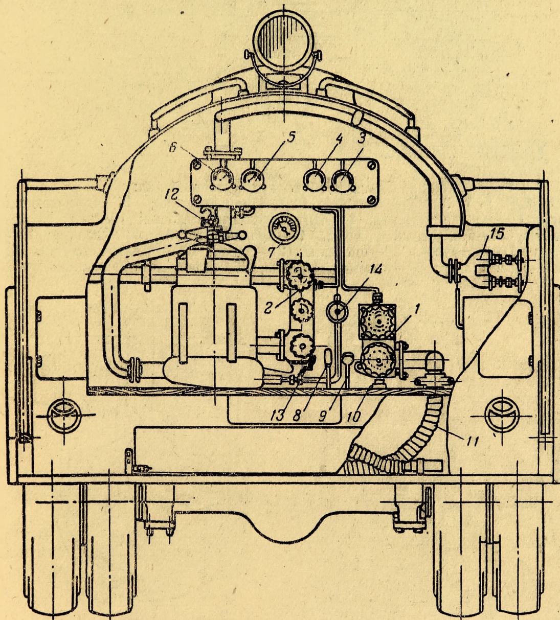
Фиг. 52. Кабина управления заправщика:
