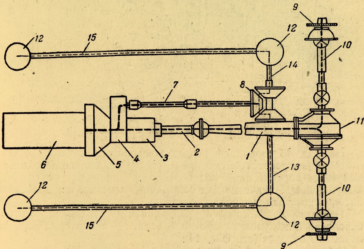
Фиг. 44. Схема расположения механизмов автолесовоза СК.
