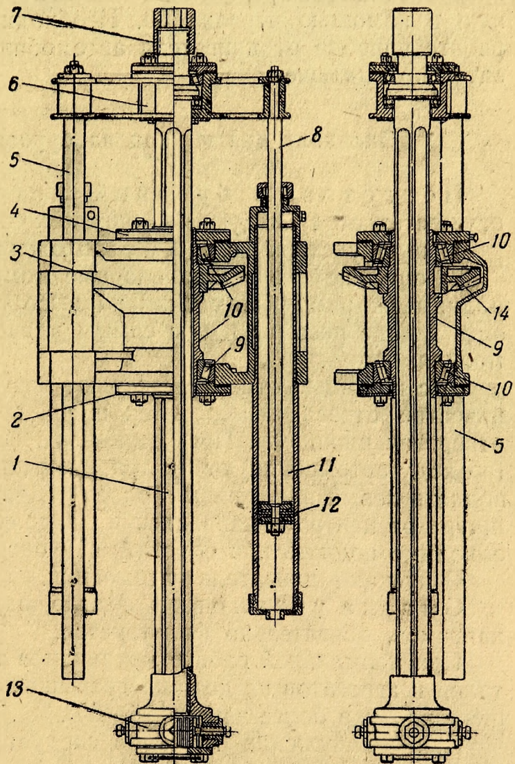
Фиг. 22. Шпиндель с механизмом привода и подачи.
