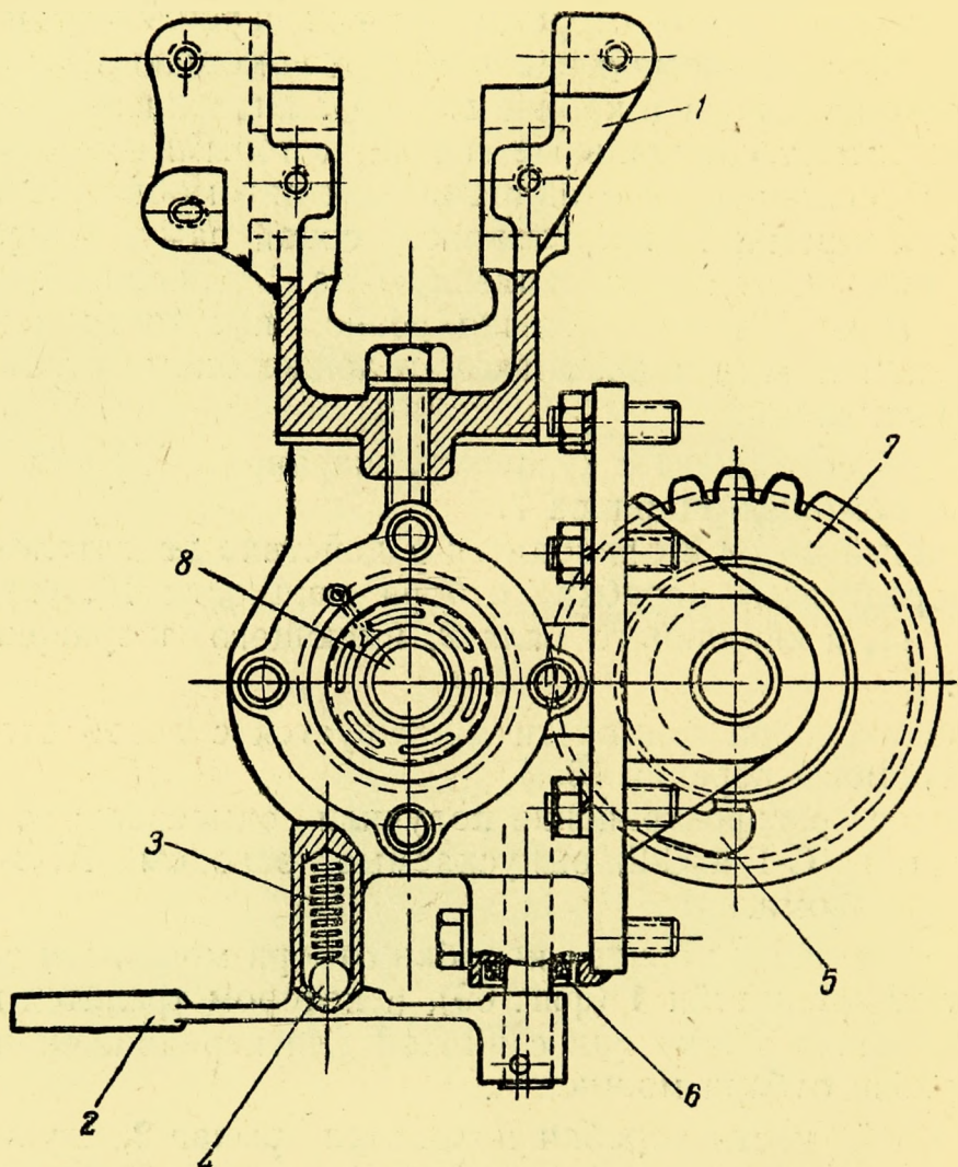
Фиг. 69. Коробка отбора мощности самосвала.
