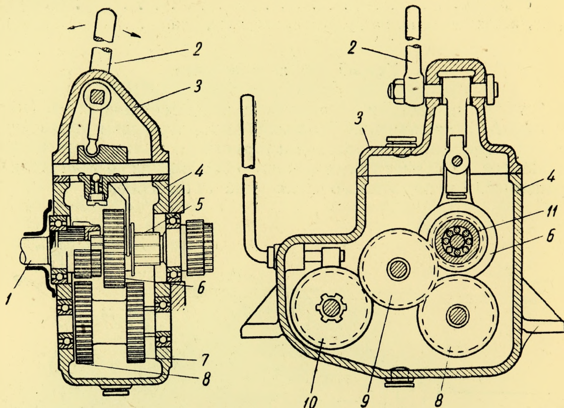
Фиг. 45. Реверсивный механизм автолесовоза СК.
