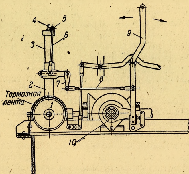
Фиг. 50. Механизм включения конуса и ограничения подъема.
