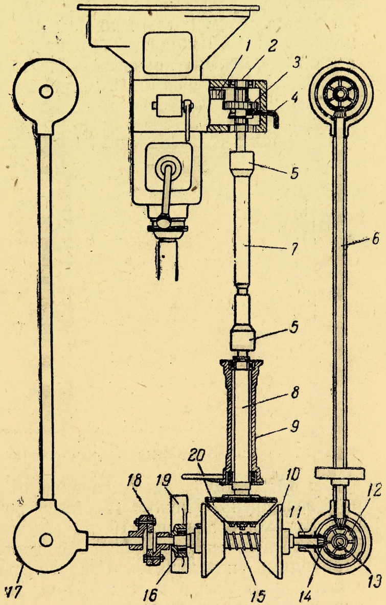
Фиг. 48. Подъемный механизм автолесовоза.
