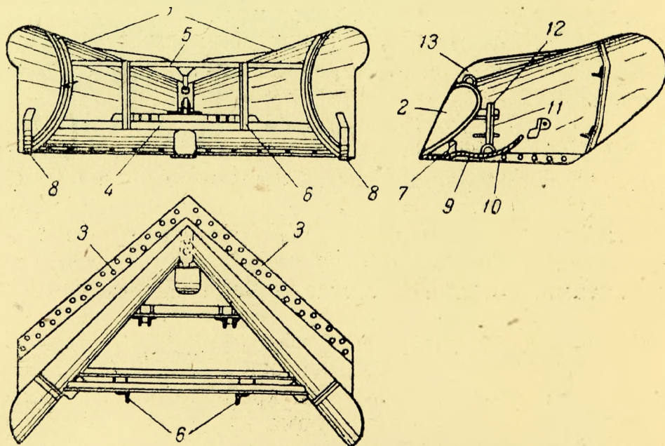
Фиг. 10. Передняя часть снегоочистителя.
