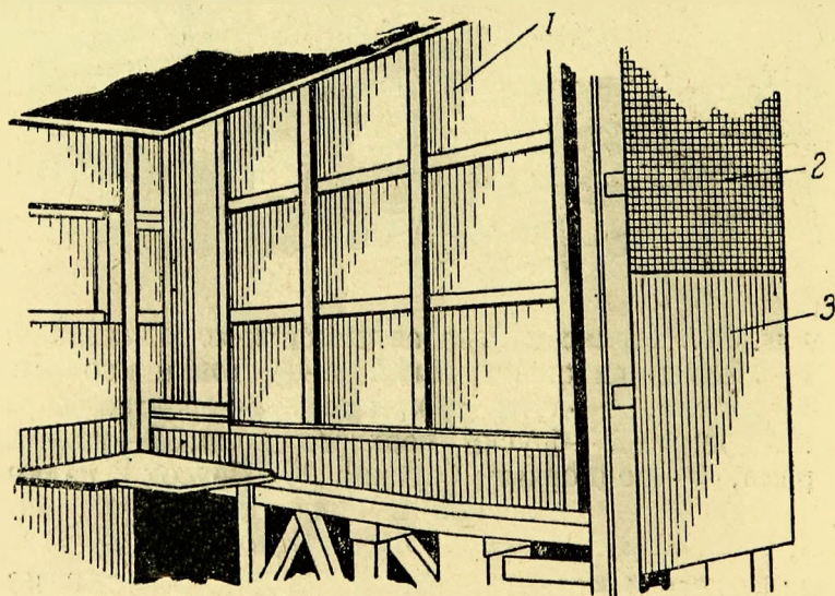
Фиг. 62. Изоляция кузова автомобиля-холодильника:
