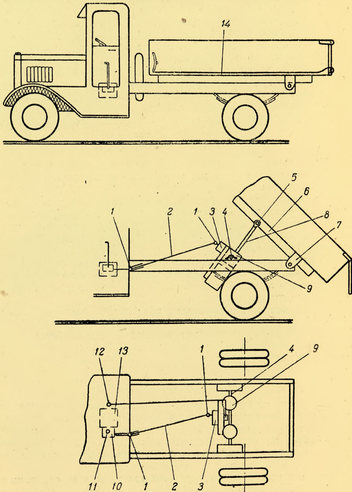
Фиг. 68. Общая схема самосвала.
