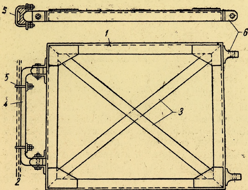
Фиг. 11. Соединительно-толкаящая рама снегоочистителя.
