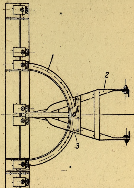
Фиг. 16. Механизм поворота отвала в горизонтальной плоскости.
