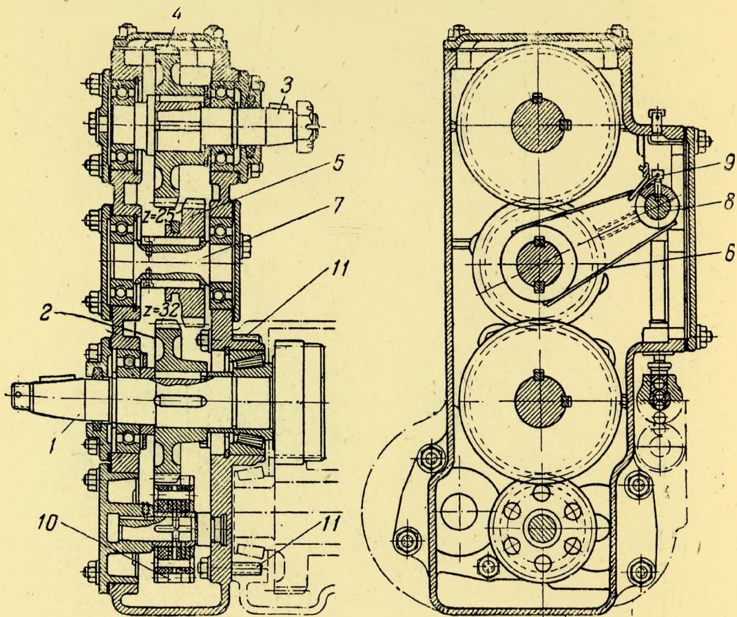
Фиг. 4. Коробка отбора мощности (разрез).
