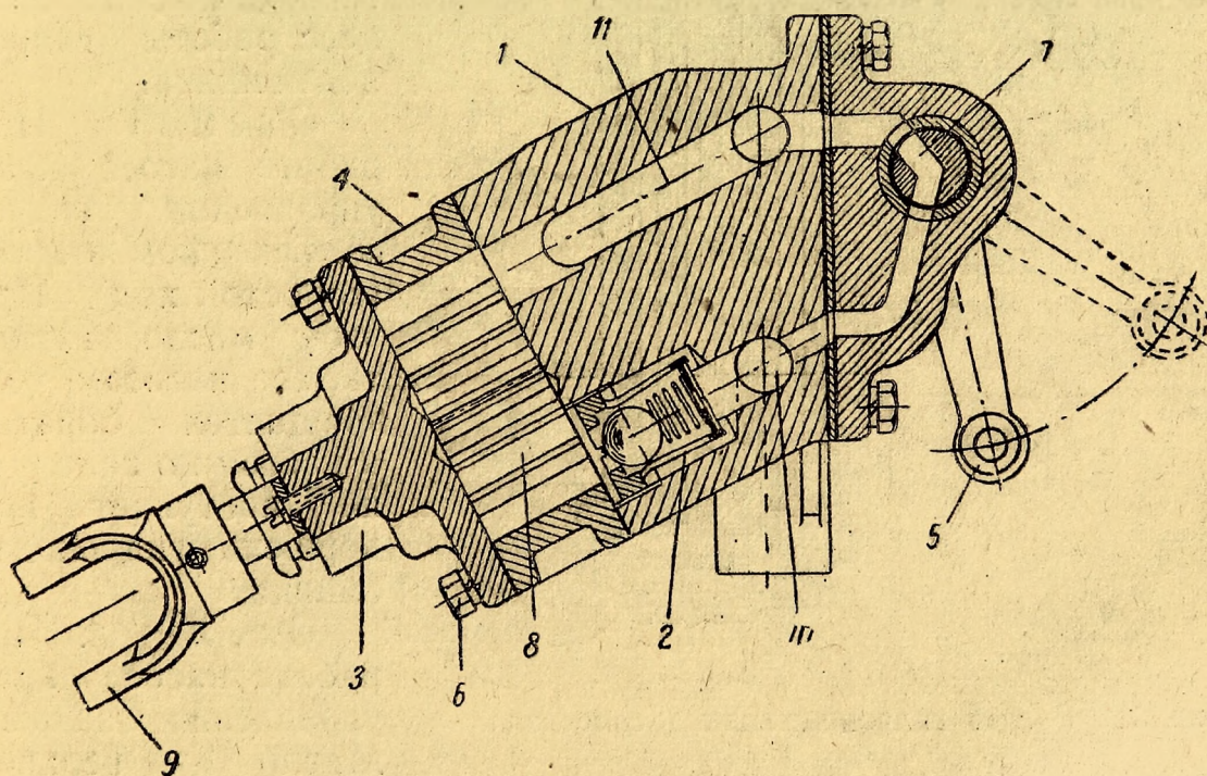
Фиг. 71. Шестеренчатый масляный насос.
