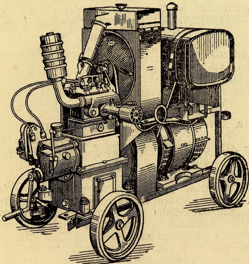
Фиг. 36. Агрегат АЛ-6/2.
