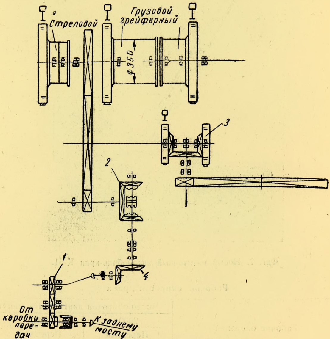
Фиг. 8. Кинематическая схема механизмов пятитонного автомобиля-крана К-51.
