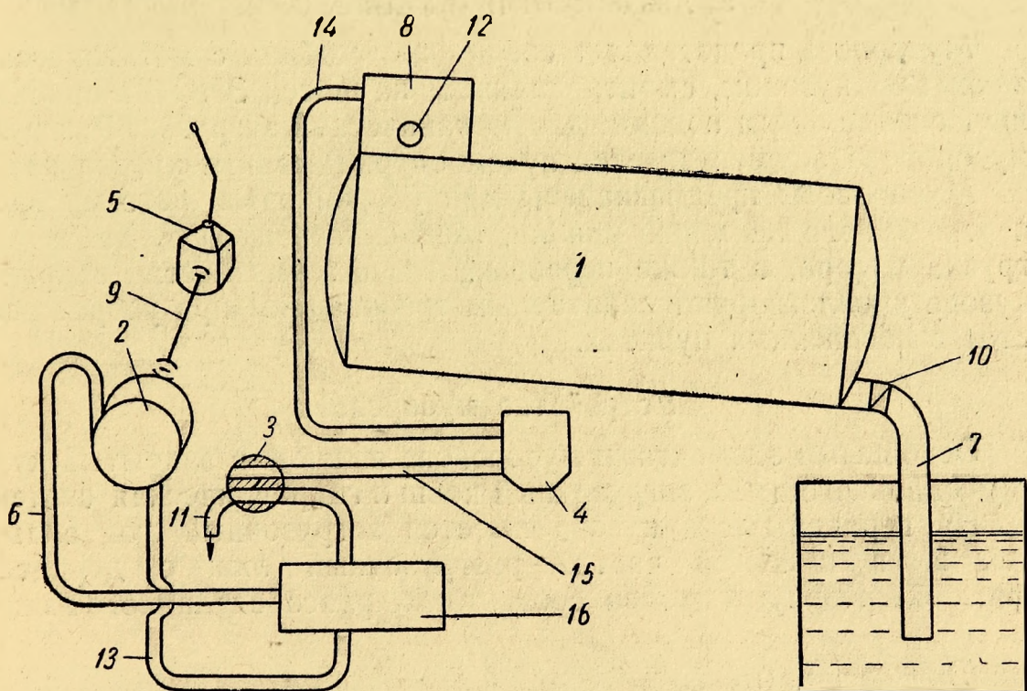
Фиг. 56. Схема устройства и работы ассенизационной автоцистерны.
