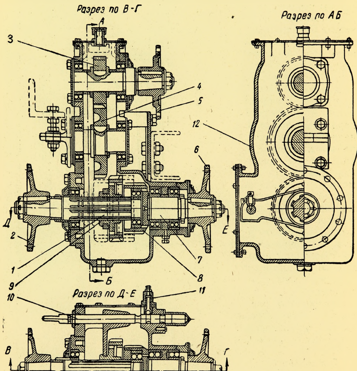
Фиг. 24. Разрез коробки отбора мощности.
