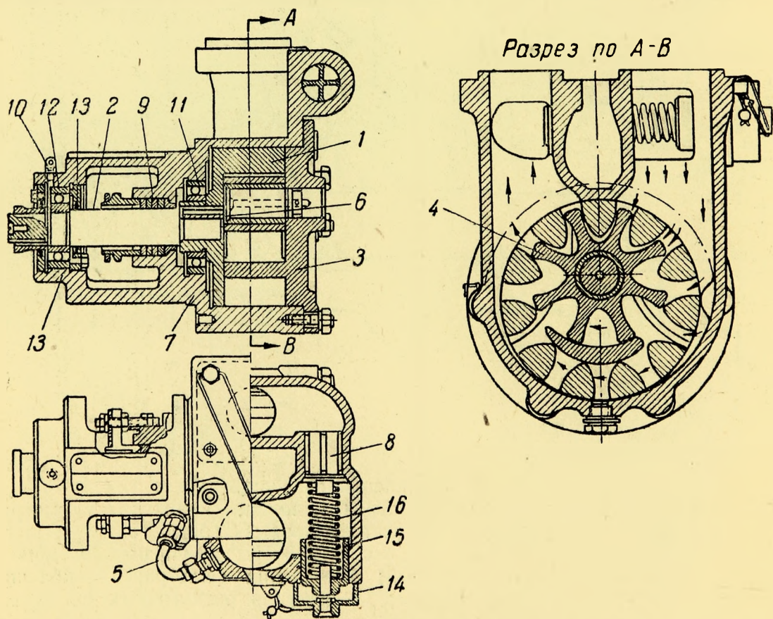
Фиг. 54. Насос заправщика:
