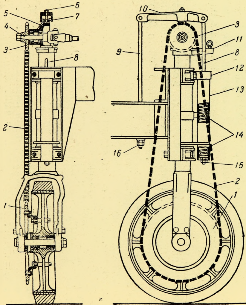
Фиг. 46. Цепная передача.
