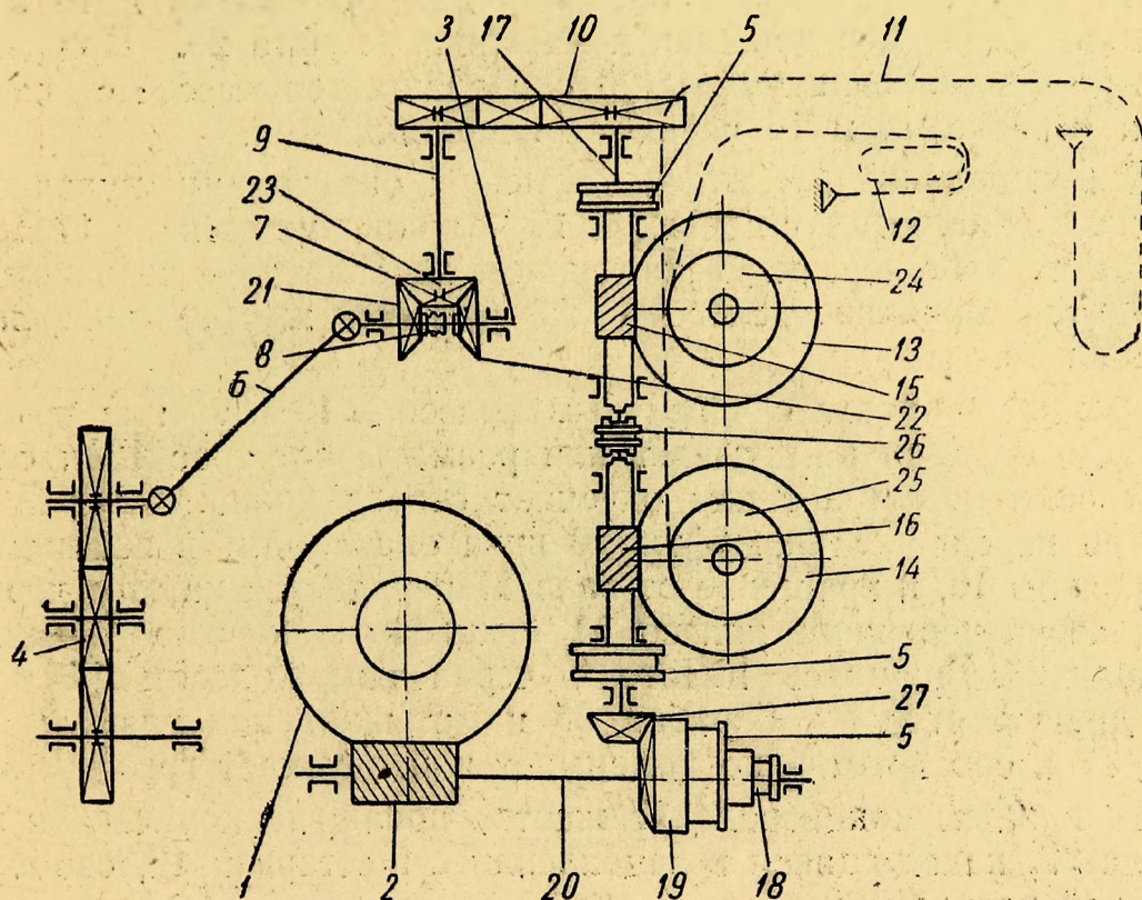
Фиг. 2. Кинематическая схема механизмов крана.
