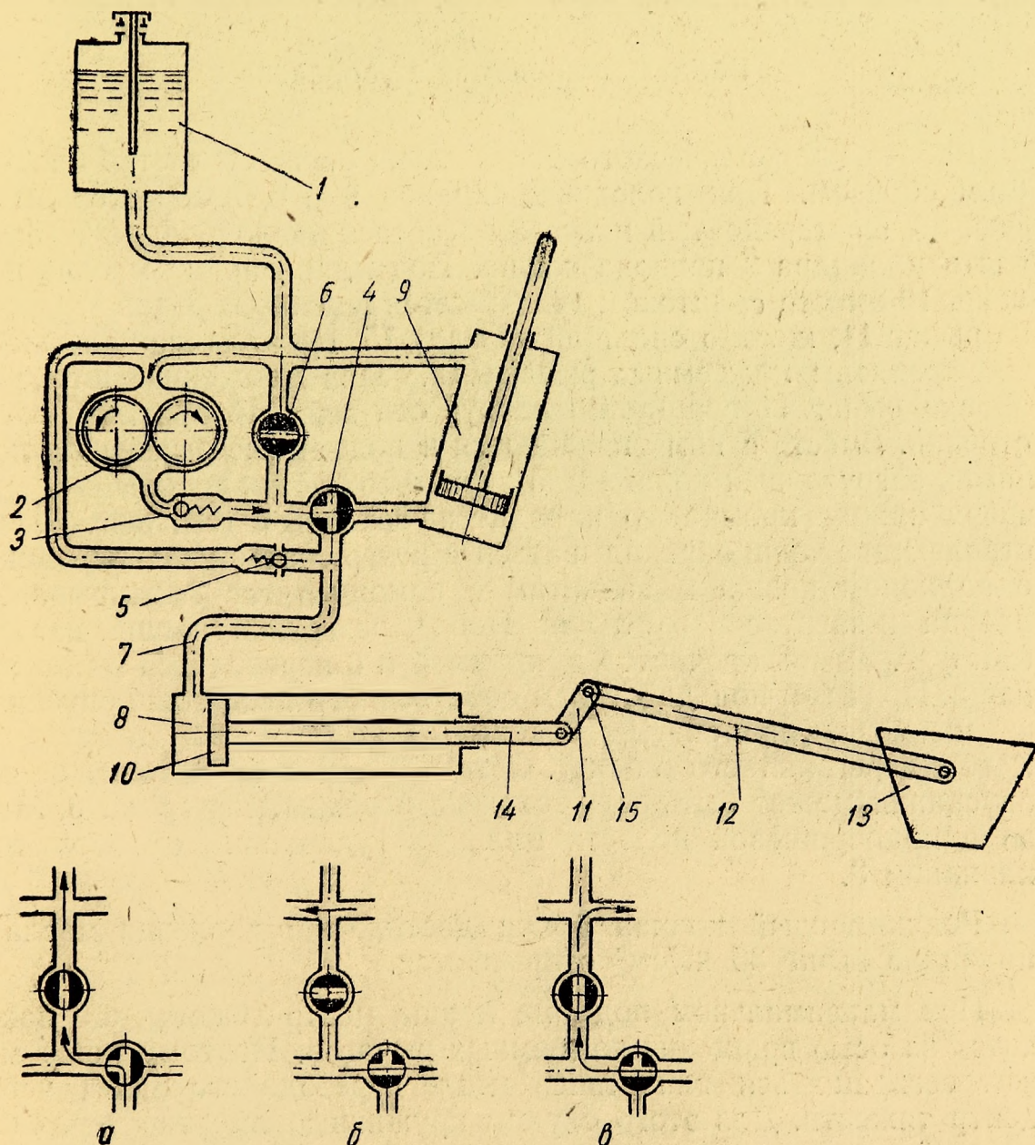
Фиг. 58. Гидравлическая схема автомобиля-мусоровоза.
