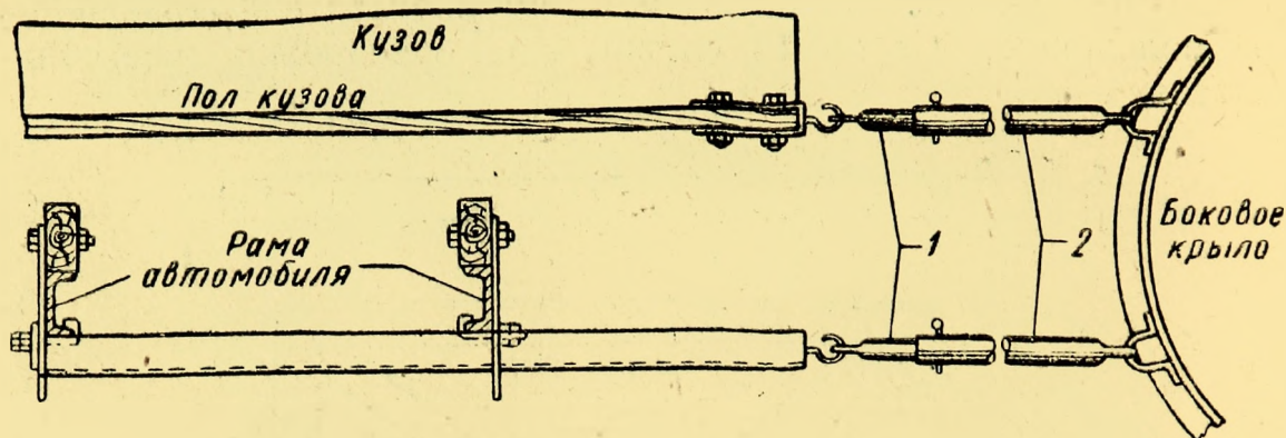
Фиг. 12. Заднее крепление бокового крыла снегоочистителя.
