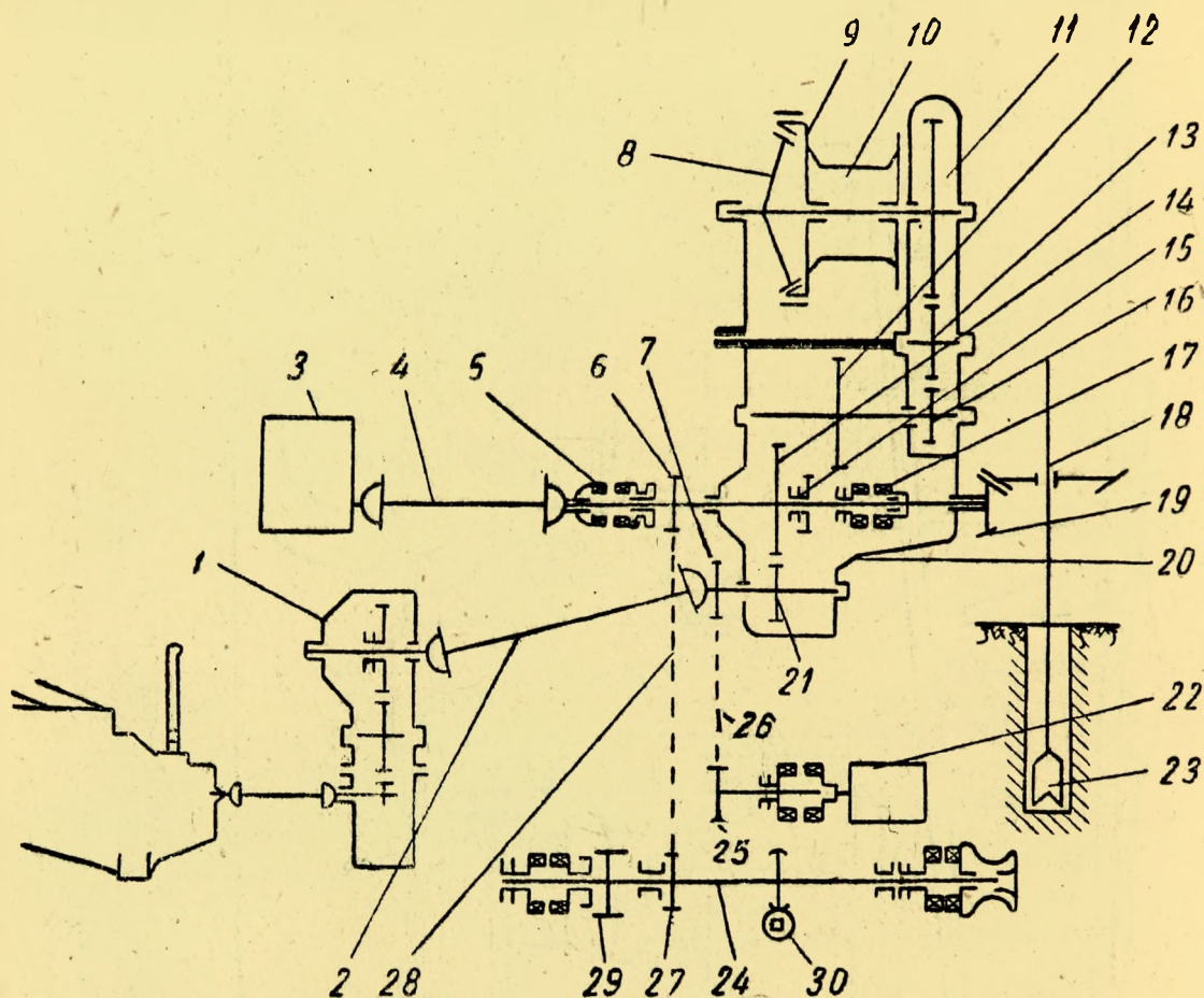
Фиг. 19. Кинематическая схема привода буровой установки.
