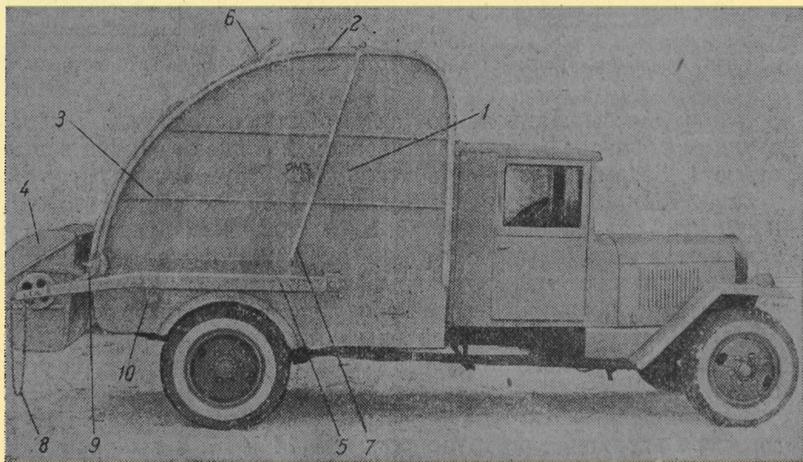
Фиг. 57. Общий вид автомобиля-мусоровоза.
