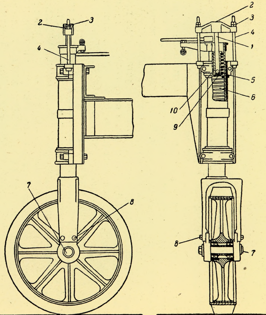
Фиг. 47. Передние колеса и амортизаторы.
