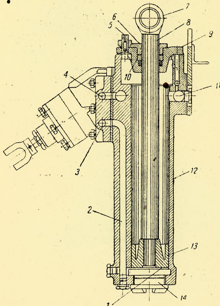
Фиг. 72. Разрез гидроподъемника самосвала.
