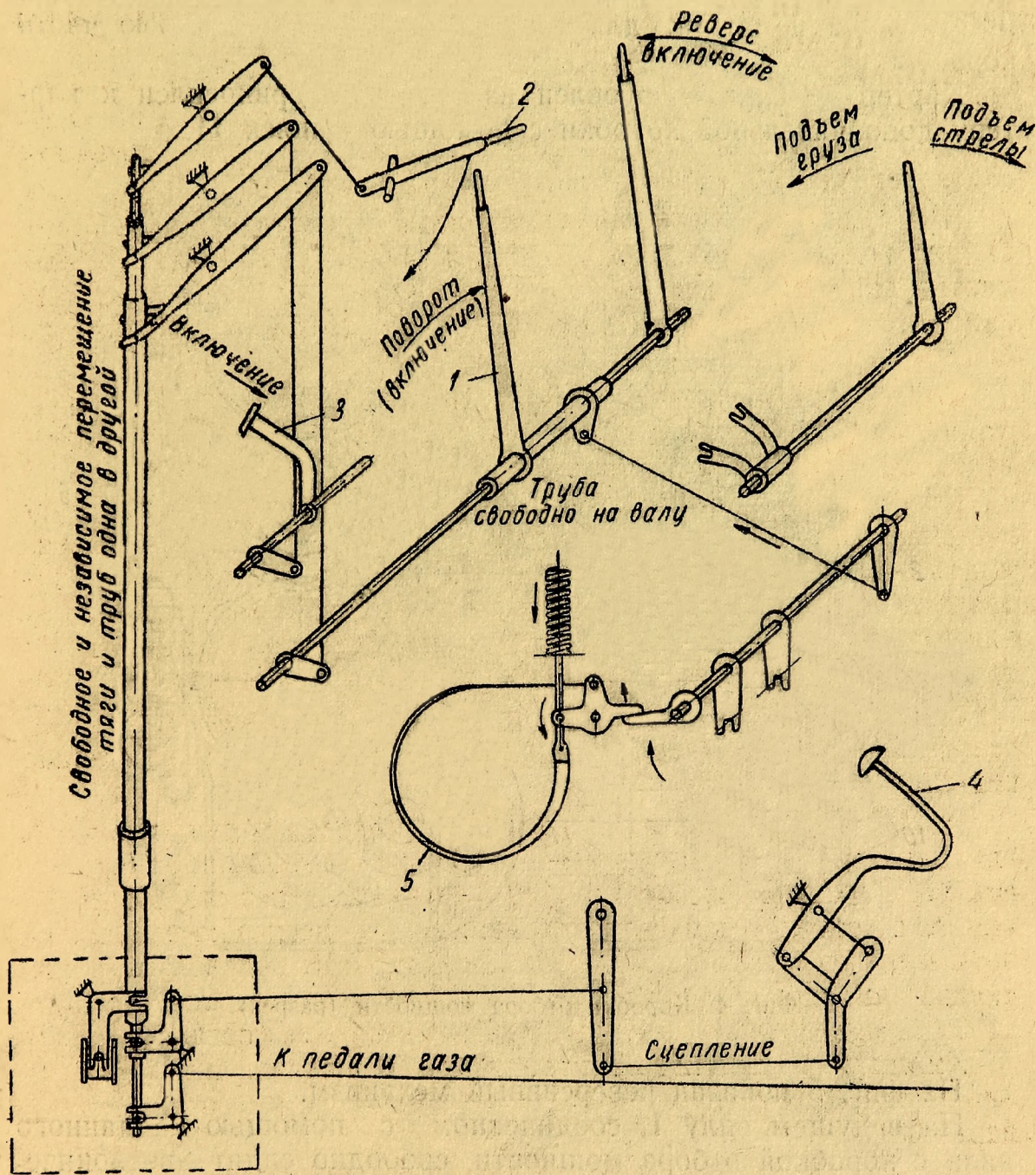
Фиг. 3. Схема управления механизмами крана:
