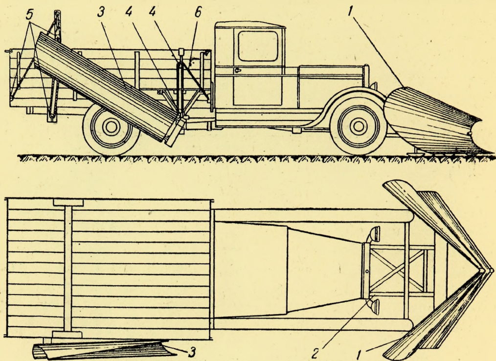
Фиг. 9. Двухотвальный снегоочиститель ДАК-5.
