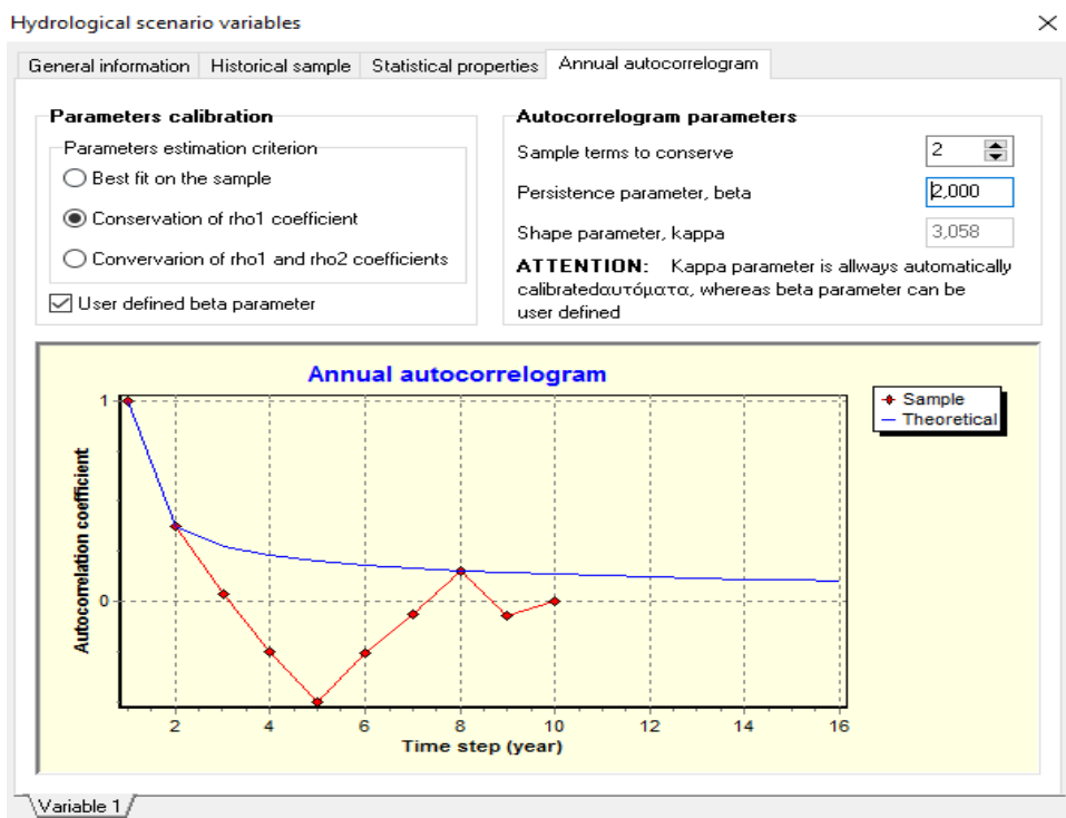
Εικόνα 5.7: Αυτοσυσχετόγραμμα απορροής
