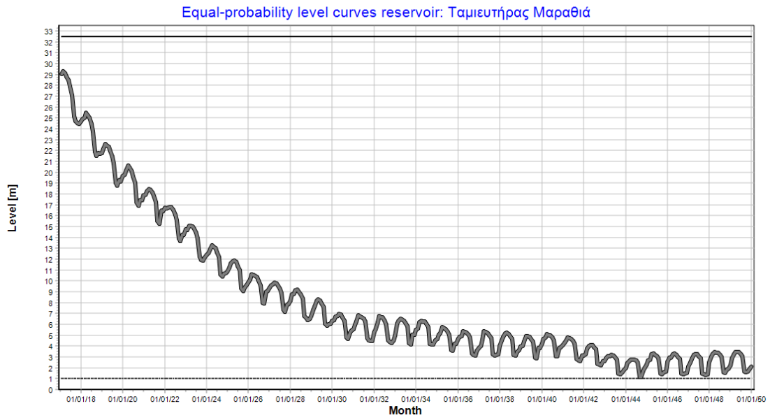
Σχήμα 6.28: Διακύμανση Στάθμης ταμιευτήρα Μαραθιά Σεναρίου 6.4.2
