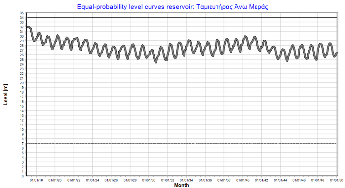
Σχήμα 6.29: Διακύμανση Στάθμης ταμιευτήρα Άνω Μεράς Σεναρίου 6.4.2
