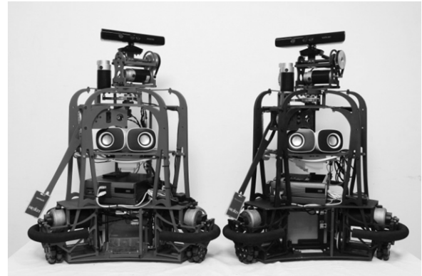
Fig. 1. Ethon robots
