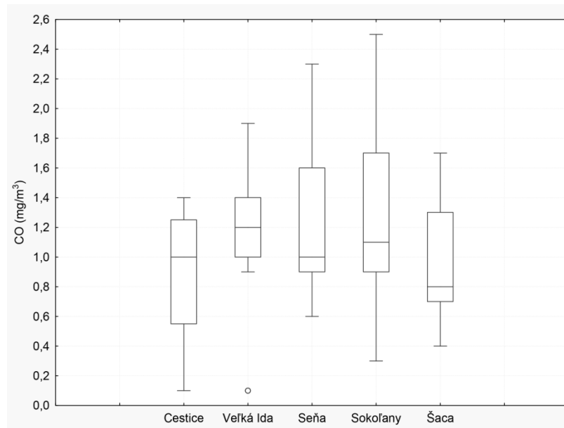
Figure 2. Carbon oxide Slika 2. Ugljični monoksid
