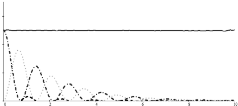
Рис. 3. Эволюция первого интеграла во времени и его компонентов: — * — — потенциальная энергия, * * * — кинетическая энергия, — — — — работа сил трения
