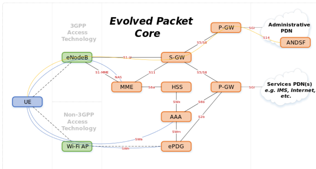
Kuva 3. 4G arkkitehtuuri. [11]
