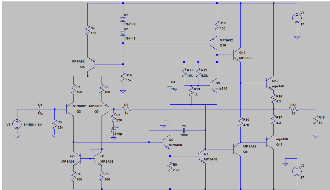
Kuva 9. Kuulokevahvistimen yhden kanavan kytkentä.
