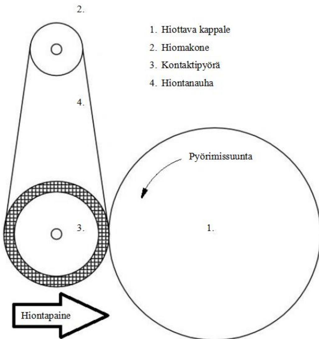
KUVIO 3. Hiomakoneen toimintaperiaate päättymättömällä nauhalla (Wintech Oy 2016)
