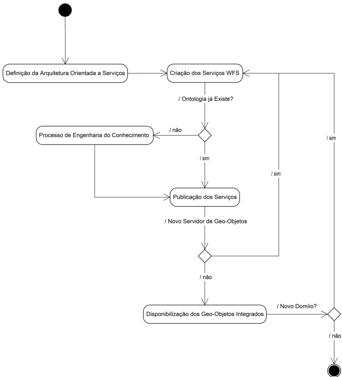
Figura 1. Diagrama de Atividades UML da Metodologia de Integração de Objetos Geográficos
