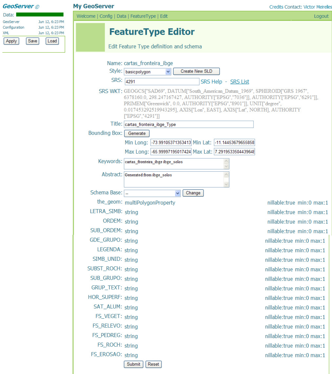
Figura 6. Publicação do Serviço no Geoserver
