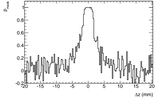
(d) p_{mask} vs. \Delta z , NTrkCut4.
