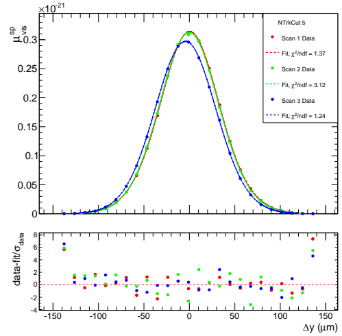
(d) y -scan, BCID 3121
