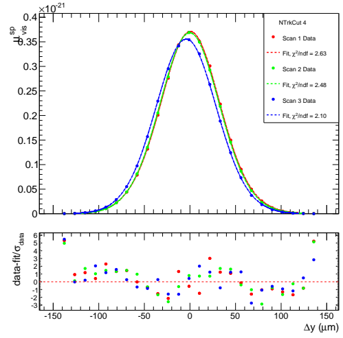
(d) y -scan, BCID 241
