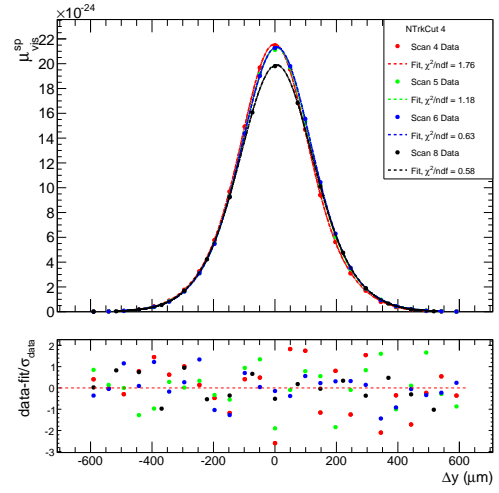
(d) y -scan, BCID 721
