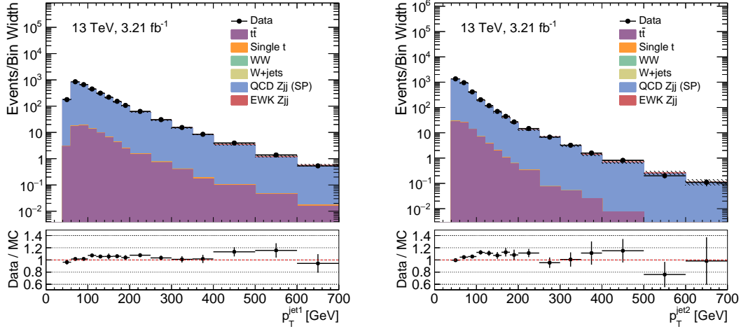
(a) p_T^{jet1} ( baseline region ).
