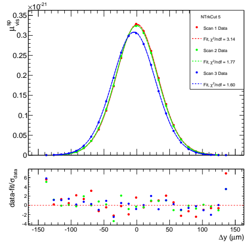
(b) y -scan, BCID 2881
