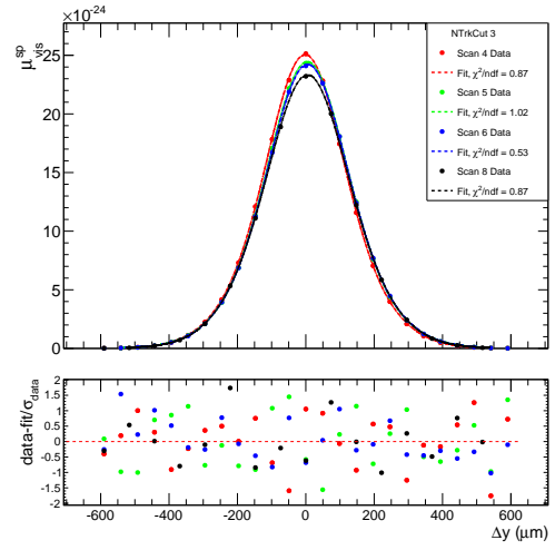
(b) y -scan, BCID 1
