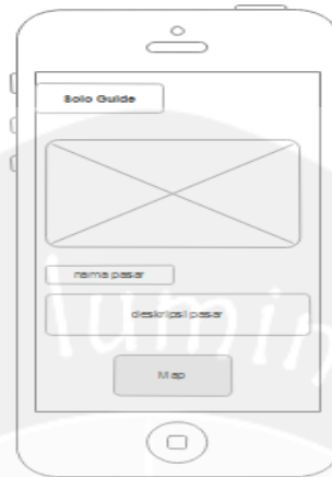
Gambar 4.7. Antarmuka Form Detail Pasar
