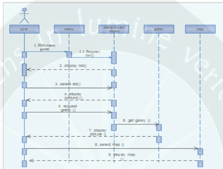
Gambar 2.2. Sequence Diagram : Fungsi Tampil Wisata
