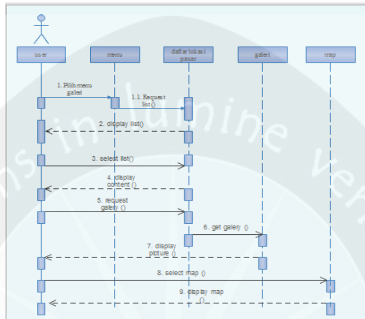
Gambar 2.4. Sequence Diagram : Fungsi Tampil Pasar
