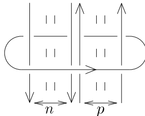
FIGURE 12. The (n, p) -tangle T^{(n,p)} .
