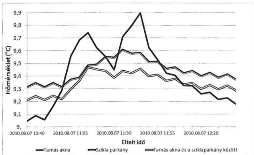
7. ábra. A csoport barlangban tartózkodásának hőmérséklet változása
