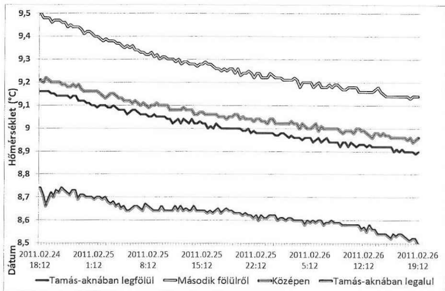
9. ábra. Tamás-aknában mért hőmérséklet
