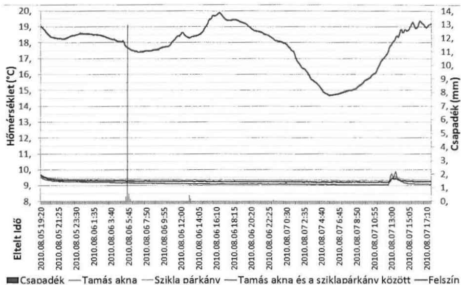
6. ábra. A Trio-barlang és felszínben mért adatok Csapadék adatok forrása: Hetvehelyi meteorológiai állomás
