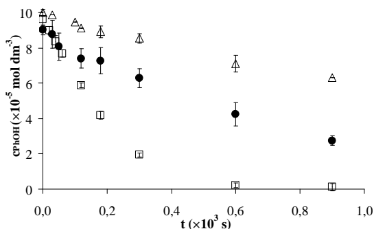
4. ábra: A PhOH VUV-fotolízise, gyöktranszferként \text{O}_2 -t ( \square ), \text{O}_2 -t és hangyasavat ( \bullet ), ill. \text{O}_2 -t és t-BuOH-t ( \Delta ) alkalmazva
