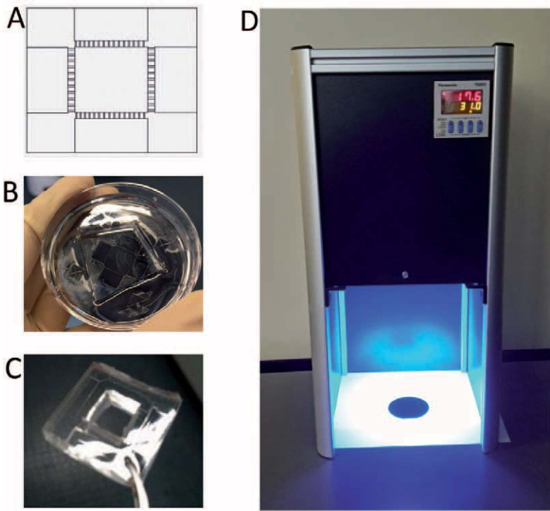
Abb. 3: A) Skizze eines beispielhaften Masken-Layouts für die Lithographie. B) Master-Wafer beim Abformungsprozess. Die Abformung lässt sich sehr oft wiederholen. C) PDMS-Replikate zur weiteren Verwendung für die Herstellung des Chips. D) Eigenbau eines „Low-Cost Mask Aligner“ mit Reinraumfunktion für die Fotolithographie.
