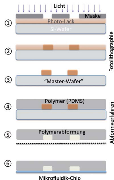
Abb. 2: A) Schematische Darstellung der Herstellungsschritte bei der „Soft Lithography“. Ein „Master-Wafer“ mit entsprechender Oberflächenstruktur wird durch Fotolithographie hergestellt. Dieser „Master-Wafer“ wird durch ein Elastomer, häufig Poly(dimethylsiloxane) abgeformt. Das PDMS-Replikat wird auf einen Träger (Glas) gesetzt, so dass Kanalstrukturen entstehen.
