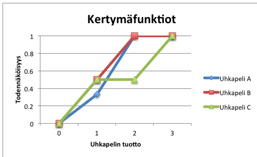
Kuva 3: Esimerkki ensimmäisen asteen stokastisesta dominanssista. Kumpikin uhkapeli A ja C dominoivat uhkapeliä B. Uhkapelin C odotusarvo on uhkapelin A odotusarvoa suurempi, mutta A ei dominoi C:tä.
