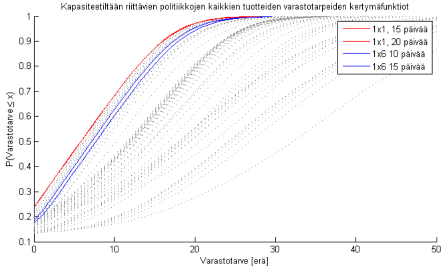
Kuva 27: Kapasiteetiltaan riittävien aikataulusmenetelmien päivittäisten varastotarpeiden kertymäfunktioit kaikkien tuotteiden osalta. Punaisella menetelmät, joita yksikään politiikka ei dominoi ensimmäisen tai toisen asteen stokastisen dominanssin mielessä.
