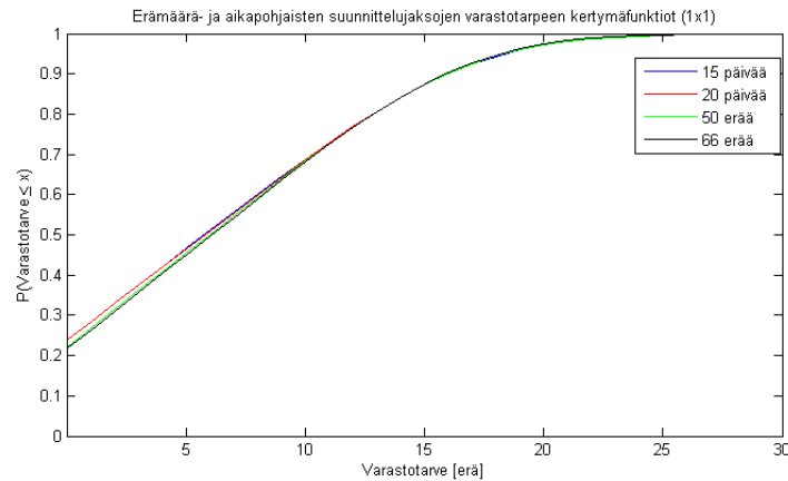
Kuva 30: Kertymäfunktiot valituista aika- ja eräperusteisista aikataulutuksen menetelmistä kaikkien tuotteiden osalta.
