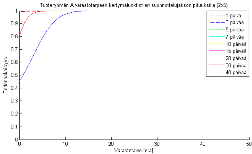
Kuva 26: Tuoteperheen A päivittäisten varastokysyntöjen kertymäfunktiot eri aikataulutuskajaksien pituuksilla. Tuotantoputken 1 minimivalmistuskoko 2 erää ja tuotantoputken 2 minimivalmistuskoko 5 erää. Kaikkien tuotteiden vastaavaan kuvaan 23 verrattuna vaaka-akselilla on kuvattu pienempi erämäärä.
