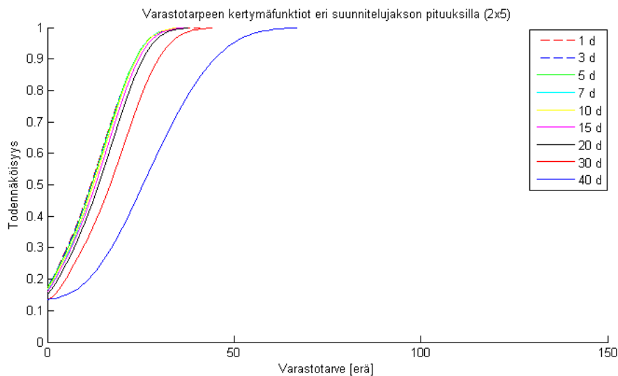
Kuva 23: Päivittäisten varastokysyntöjen kertymäfunktiot eri aikataulutuskantojen pituuksilla. Tuotantoputken 1 minimivalmistuskoko on 2 erää ja tuotantoputken 2 minimivalmistuskoko on 5 erää.
