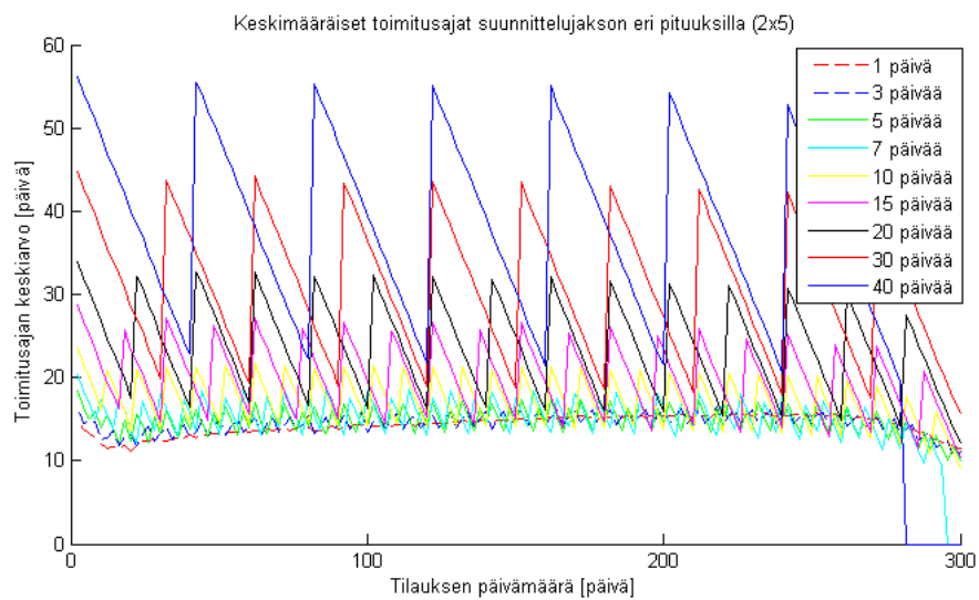
Kuva 17: Tuote-erien keskimääräiset toimitusajat tilauspäivämäärän mukaisesti eri aikataulutuskajsojen pituuksilla. Tuotantoputken 1 minimivalmistuskoko on 2 erää ja tuotantoputken 2 minimivalmistuskoko on 5 erää.
