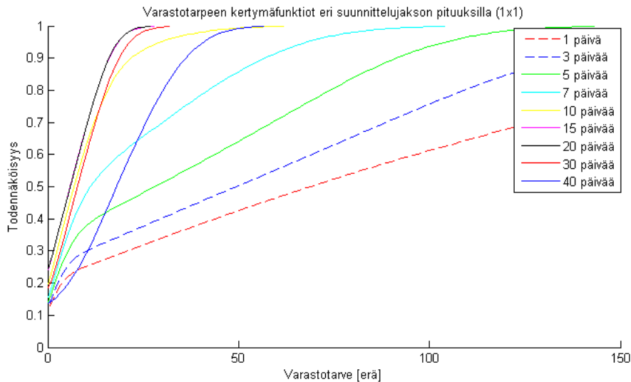
Kuva 21: Päivittäisten varastokysyntöjen kertymäfunktioita eri aikataulutussuunnitelmissa. Tuotantoputkissa 1 ja 2 ei ole minimisarjapituusvaatimuksia.
