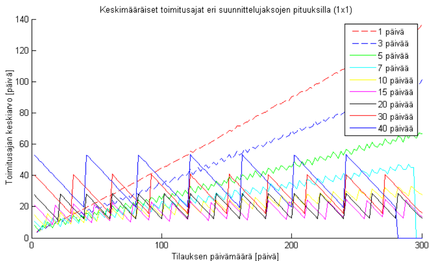
Kuva 15: Tuote-erien keskimääräiset toimitusajat tilauspäivämäärän mukaisesti eri aikataulutusjaksojen pituuksilla. Tuotantoputkien aikataulutuksessa ei minisarjapituuksia.
