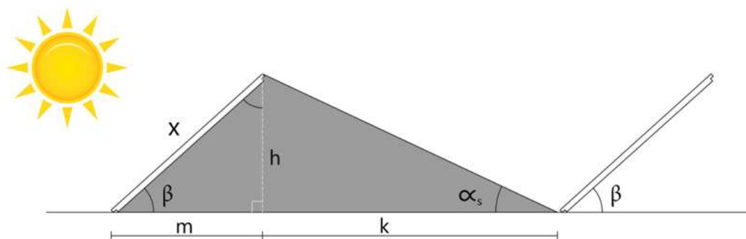
Kuva 14. Aurinkosähköpaneelirivien vähimmäisetäisyys
