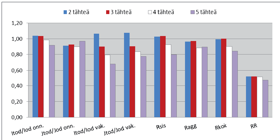
Kuva 40 Tutkittaville automalleille saadut havainnot EuroNCAP-tähtien avulla ryhmiteltynä. Riskilukujen keskiarvoja eri automalleilla, missä Rsis, Ragg, Rkok ja RR ovat kuvaavat absoluuttista loukkaantumiseriskää. I kuvaa loukkaantumisia tarkasteltavassa automallissa ja J onnettomuuden vastapuolen loukkaantumisia. tod tarkoittaa havaittuja loukkaantumisia ja od laskentamenetelmän antamia odotusarvoja. Riskivertailut sisäisen turvallisuuden ja aggressiivisuuden osalta on esitetty sekä onnettomuusmääriin että vakuutusvuosiin pohjautuvilla odotusarvoilla.
