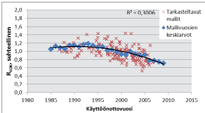
Kuva 15 Käyttöönottovuoden yhteys automallin kokonaisvammauttavuus kahden henkilöauton välisissä törmäyksissä. [vamm. kulj./ 100 onn.]. Siniset neliöt ovat mallivuosien keskiarvoja ja punaiset ristit tarkasteltavia automalleja. Aineisto vuosilta 2001–2009.
