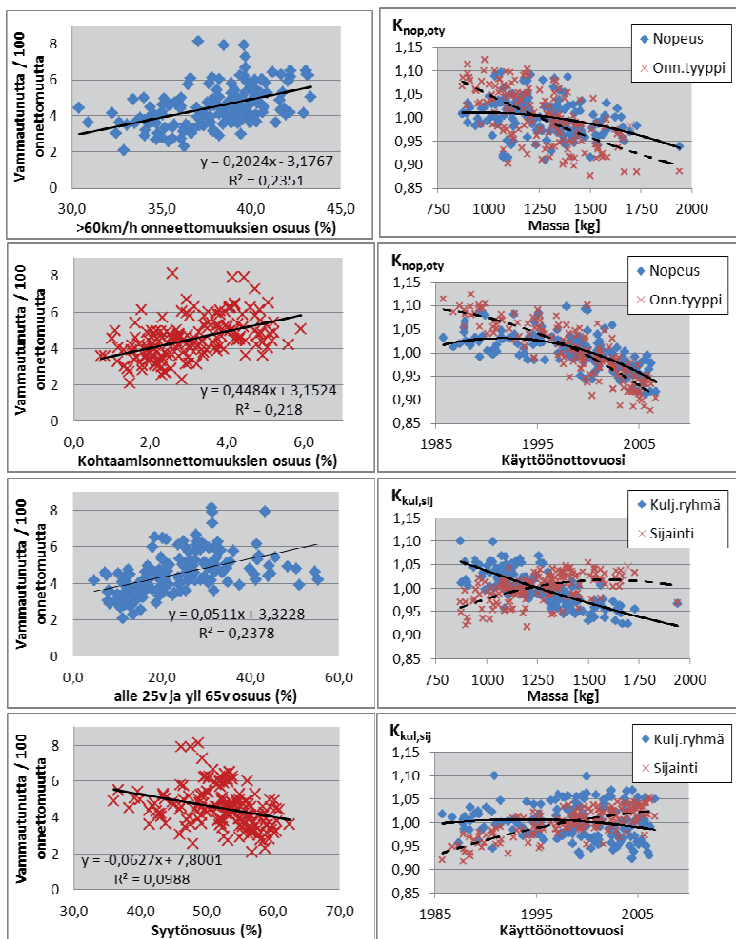
Kuva 41 Autosta riippumattomien tekijöiden yhteys kuljettajan vammautumisriskiin kahden henkilöauton välisessä onnettomuudessa sekä kertoimien yhteys auton massaan ja käyttöönottovuoteen. Onnettomuus aineisto vuosilta 2001–2009.
