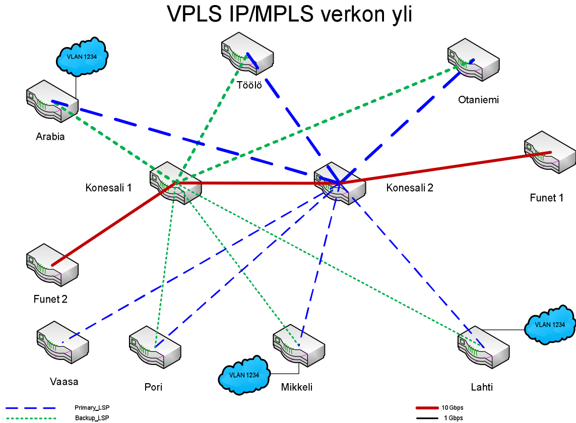
Kuva 6 VPLS IP/MPLS verkon yli
