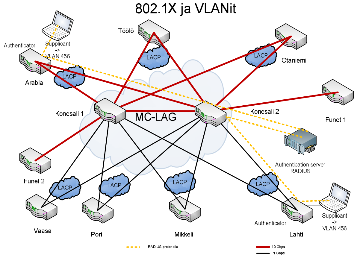
Kuva 12 802.1X porttiantentikointi
