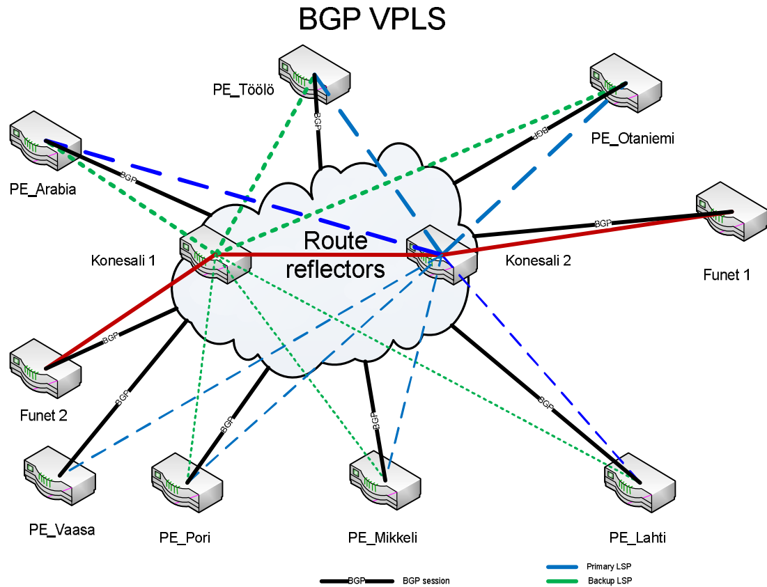
Kuva 8 BGP VPLS
