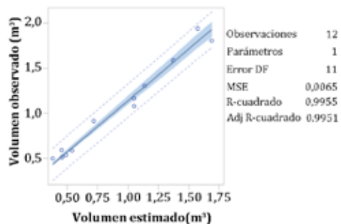
Figura 2. Volumen observado y estimado sin corteza para E. nitens , en suelos de cenizas volcánicas.
