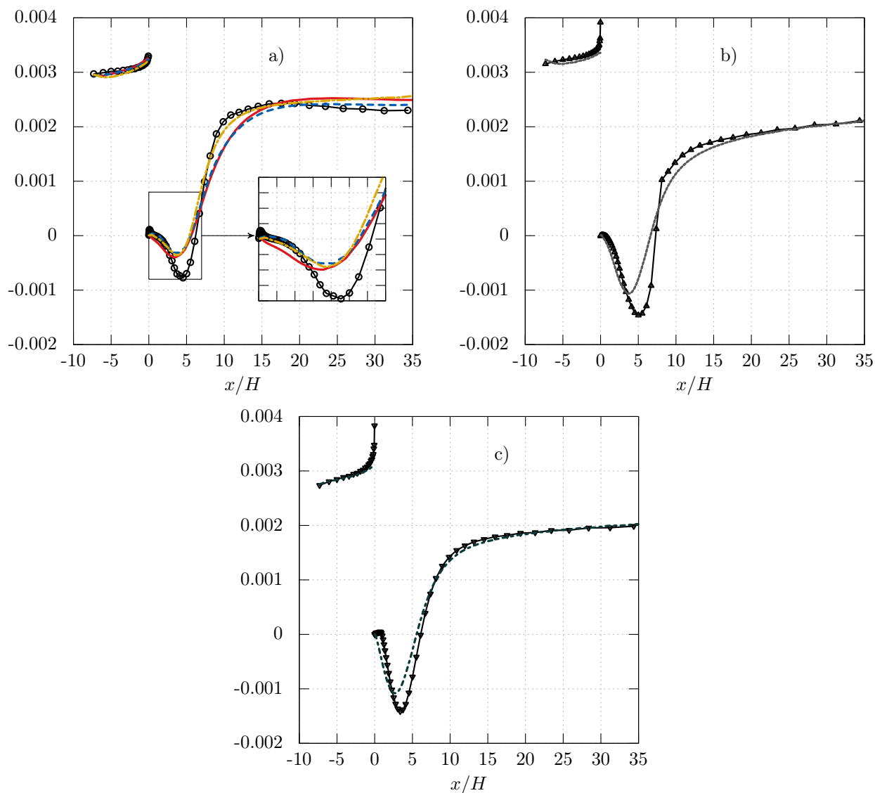
FIGURE 4.25 – Coefficient de frottement C_f pour a) : EB-RSM en adhérence ( —○— ) et lois de paroi AAWF ( — ), ASWF ( - - - ) et « scalable wall functions » SSG ( - · - · - ), b) : Bl-v^2-k en adhérence ( —▲— ) et lois de paroi AdWF ( ····· ), c) : k-\omega -SST en adhérence ( —▼— ) et lois de paroi standard ( ····· ).
