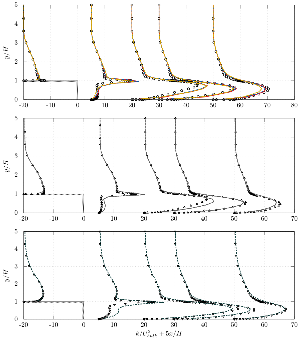
FIGURE 4.27 – En haut : Calcul EB-RSM en adhérence ( \circ ) et lois de paroi AAWF ( — ), ASWF ( - - - ) et « scalable wall functions » SSG ( - - - ). Au milieu : Calcul Bl-v^2-k en adhérence ( \blacktriangle ) et lois de paroi AdWF ( ..... ). En bas : Calcul k-\omega -SST en adhérence ( \blacktriangledown ) et lois de paroi standard ( - - - ).
