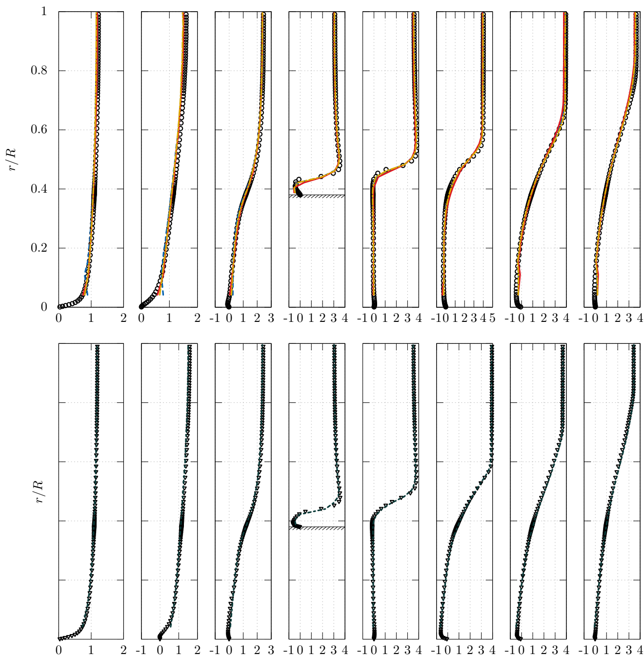
FIGURE 5.10 – Profils de vitesse U/U_b pour En haut : Calcul EB-RSM en adhérence ( \text{---}\circ\text{---} ) et lois de paroi AAWF ( \text{---} ), ASWF ( \text{- - -} ) et « scalable wall functions » SSG ( \text{- . - .} ). En bas : Calcul k\text{-}\omega\text{-SST} en adhérence ( \text{---}\blacktriangledown\text{---} ) et lois de paroi standard ( \text{. . . . .} ).
