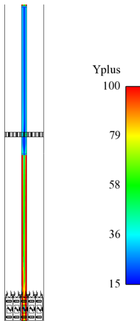
FIGURE 1.4 – Distance adimensionnelle à la paroi autour du tube central à travers deux grilles (assemblage combustible 5 \times 5 ).
