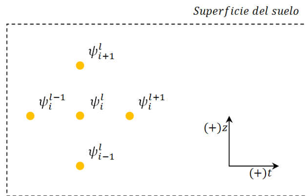
Figura 2: Discretización del dominio
