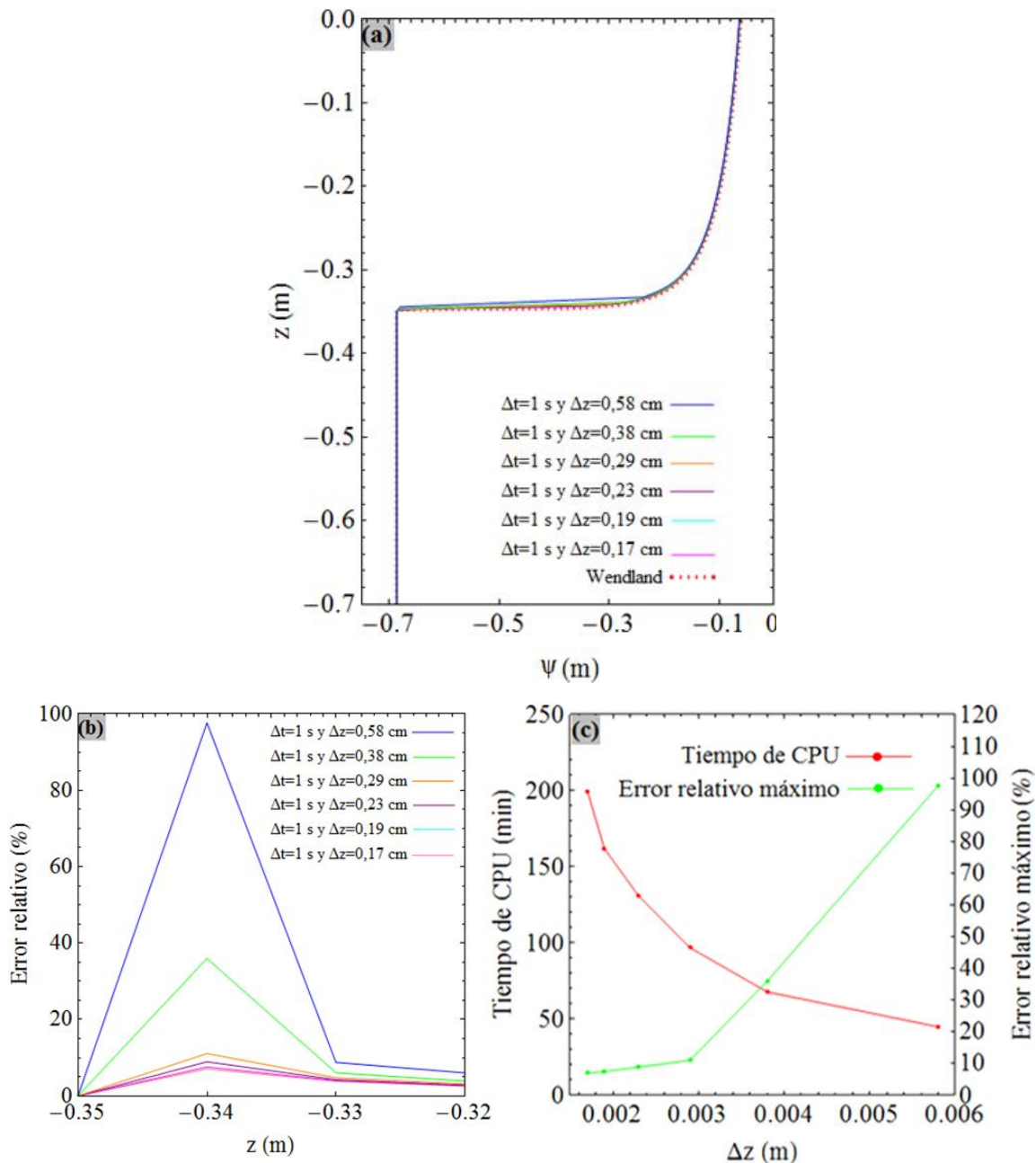
Figura 8: (a) Perfil de cantidad de agua para 1,75 horas con datos de la segunda aplicación ( \Delta t = 1 s para distintos valores de \Delta z ) (b) Error relativo máximo para distintos valores de \Delta z . (c) Tiempo de CPU y error relativo máximo para diferentes valores de \Delta z
