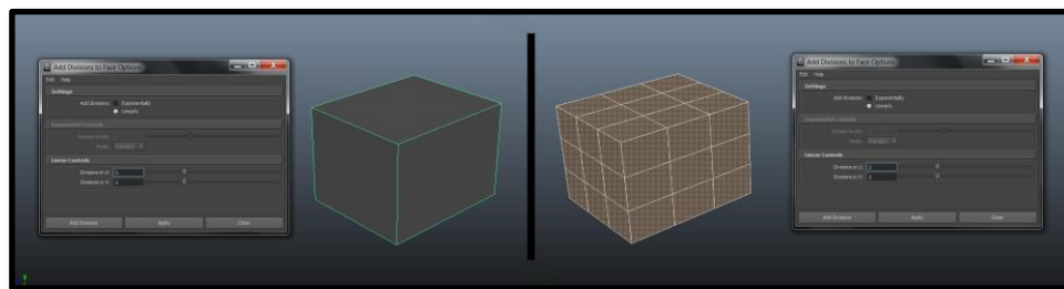
Slika 2.4 Dodavanje divizija
