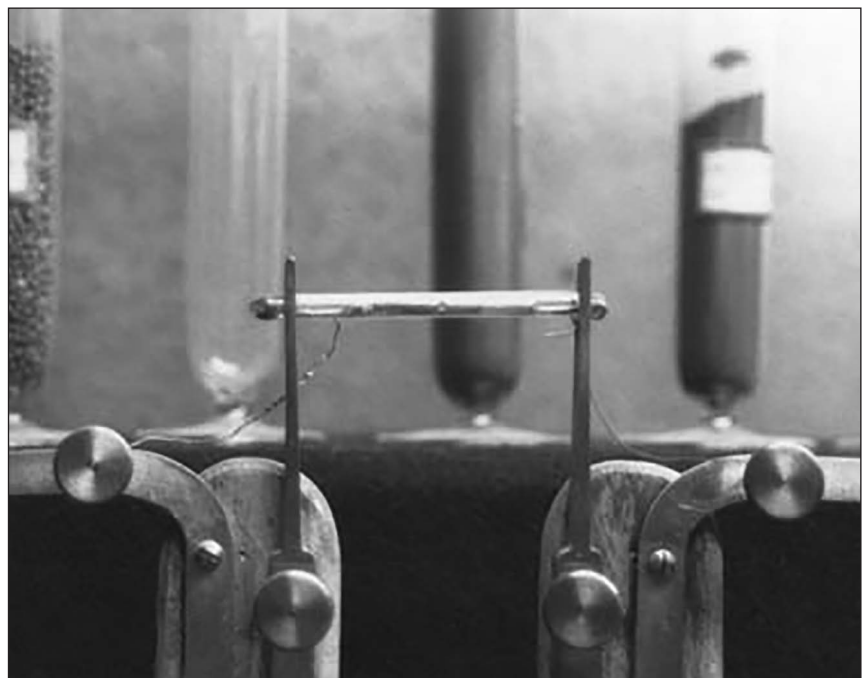
FIGURE 1 – One of Branly’s early radioconducteur , 1890. (Photo courtesy of Wikimedia Commons.)
