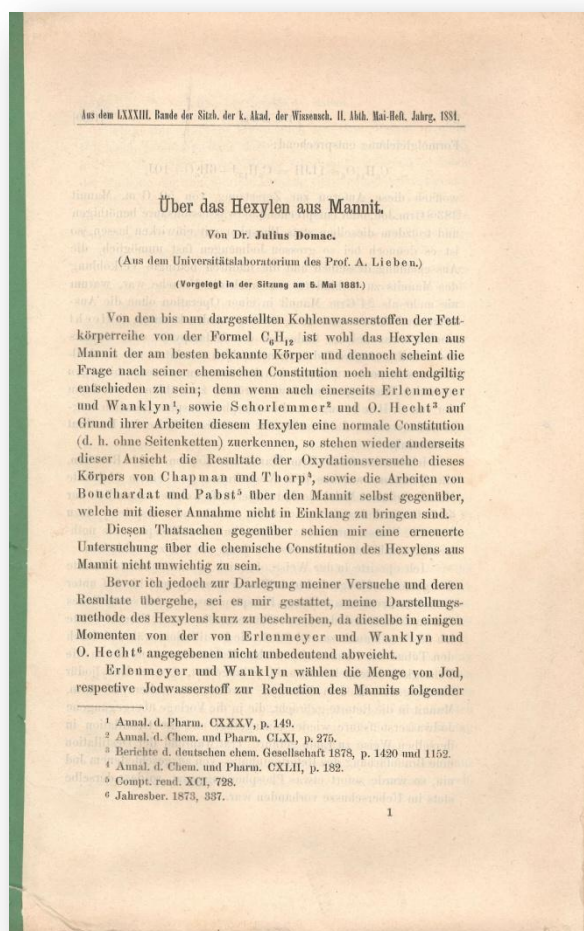
Slika 46 Naslovnica Domčevog rada Über das Hexylen aus Mannit ( O heksilenu iz mannita ) objavljenog u Izvyješću Carske akademije znanosti u Beču i časopisu Monatshefte für Chemie , Beč, 1881. (GMVkB B2)
