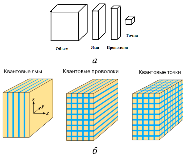
Рисунок 1.12 – Последовательность прямоугольных наноструктур (а) и геометрические области квантования в квантоворазмерных структурах (б)
