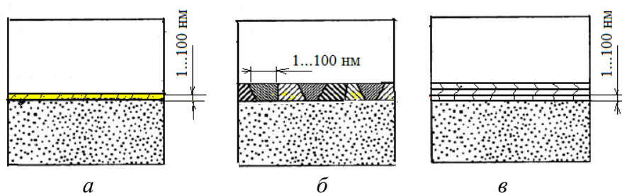
Рисунок 1.10 – Наноструктурные покрытия: a – нанослойные; б – нанокристаллические; в – многослойные
