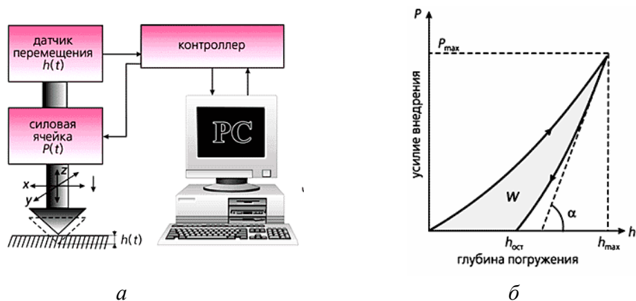
Рисунок 1.4 – Принципиальная схема нанотестирования поверхности (а) и типичная диаграмма «сила-перемещение» при наноиндентировании – аналог диаграммы \sigma - \varepsilon в традиционных макроиспытаниях (б): h_{\max} – максимальная глубина внедрения индентора; h_{\text{ост}} – глубина отпечатка, оставшегося после снятия нагрузки; W – поглощенная энергия
