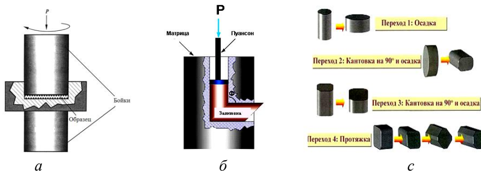
Рисунок 1.28 – Основные методы ИПД:
