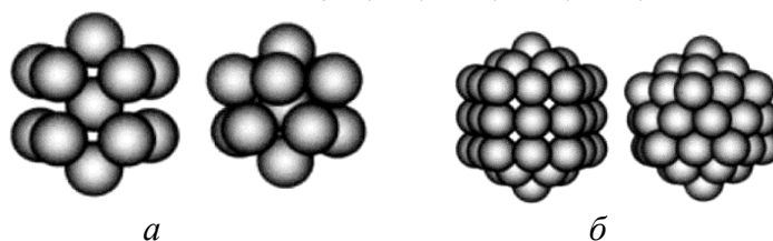
Рисунок 1.9 – Атомные кластеры с числом атомов («магическими» числами) 13 (а) и 55 (б)
