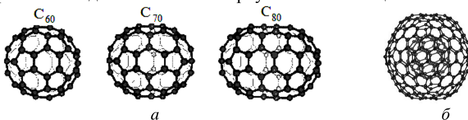
Рисунок 1.24 –Примеры структур на основе углеродных кластеров: a – фуллерены C_{60} , C_{70} , C_{80} ; б – многослойный фуллерен C_{60}/C_{240}
