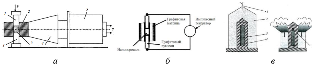
Рисунок 1.27 – Схемы методов динамического прессования: а – установка для ультразвукового прессования: 1 – пуансон; 2 – матрица; 3 – заготовка; 4 – УЗ-концентратор; 5 – магнитострикционный преобразователь, соединенный с УЗ-генератором; б – агломерация пульсирующим электрическим током; в – схема взрывного компактирования: 1 – электродетонатор; 2 – заряд взрывчатого вещества; 3 – прессуемый порошок; 4 – ампула; 5 – спрессованный порошок (компакт)
