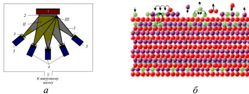
Рисунок 1.11 – Схема установки молекулярно-лучевой эпитаксии (а) и схема роста пленки путем «атомной укладки» (б):
