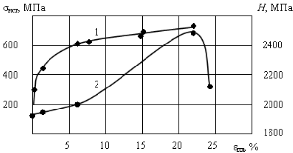
Рис. 6. – Зависимость \sigma_{ист} (кривая 1) и микротвердости (кривая 2) от пластической деформации растяжением образцов из стали 30X15
