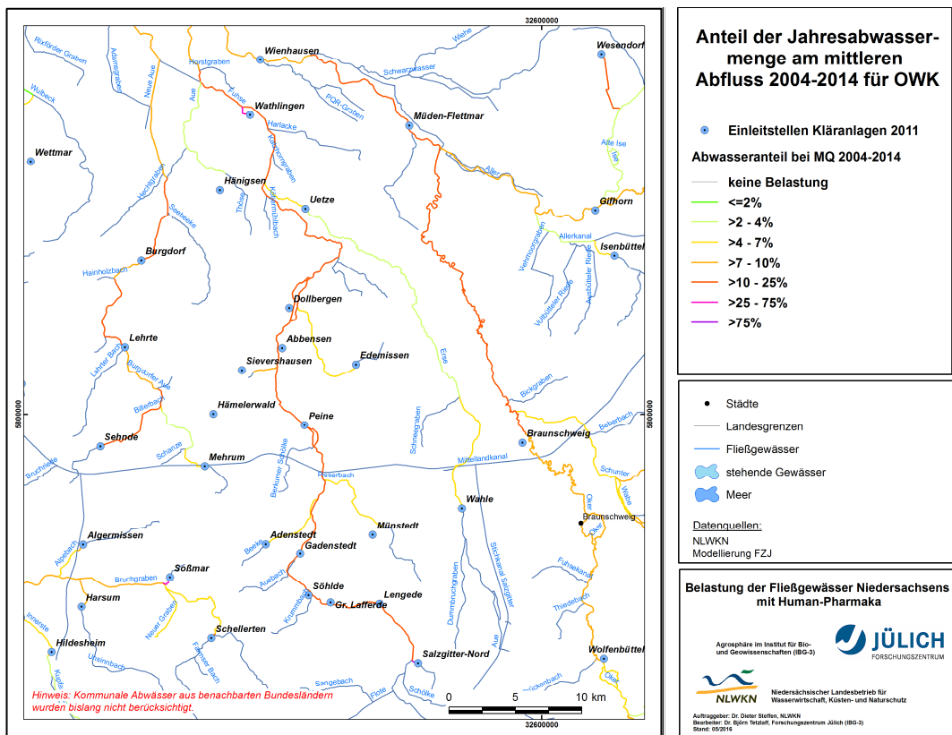
Abbildung 4-9: Ausschnittsvergrößerung der Belastungsregion Fuhse-Oker
