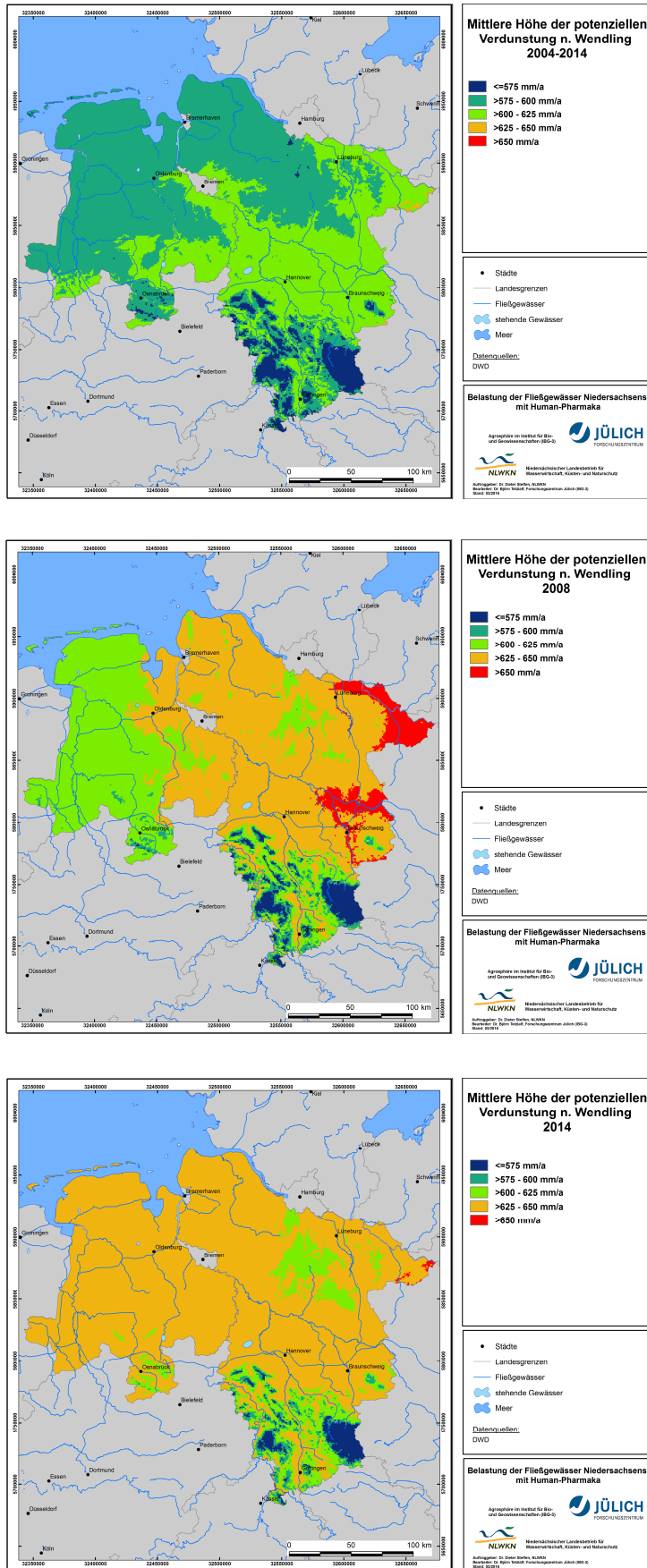
Abbildung 3-9: Karte der mittleren potenziellen Verdunstungshöhe
