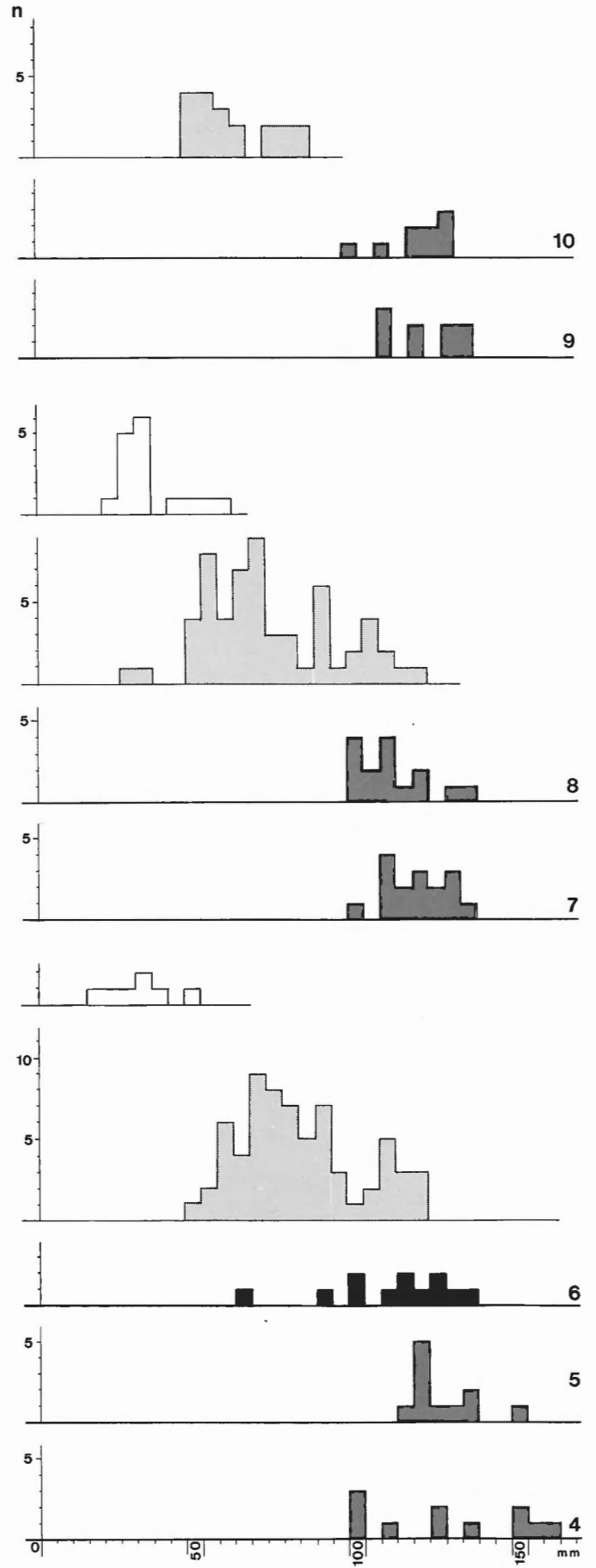
Abb. 23: Lattigen VI-Riedstation Durchmesser der Pfähle einzelner Strukturen des Schlagjahres 3391 v.Chr. Schwarz = Häuser 4-10, Raster = flankenseitige und umlaufende Pfahlreihen, weiss = landseitige Pfahlreihen.
