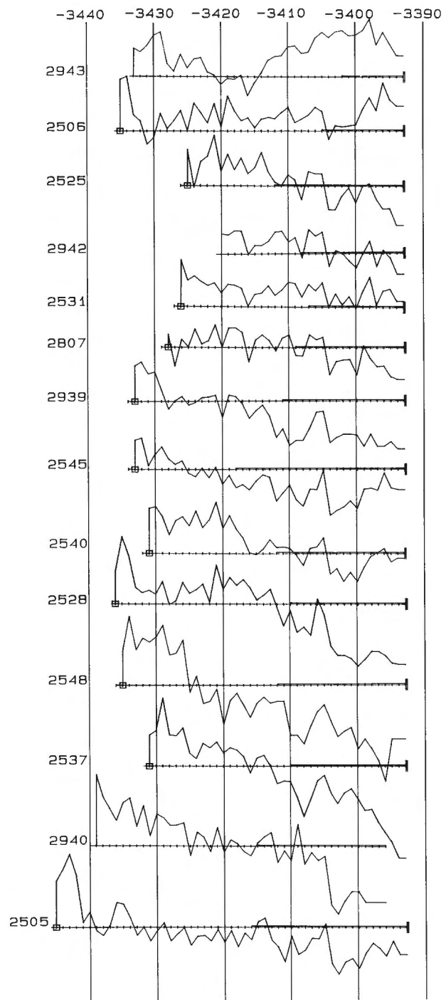
Abb. 36: Latrigen VI-Riedstation. Dendrochronologische Messkurven zu den Pfählen des Hauses 1 (links) und den dazugehörigen Pfahlreihen (rechts).
