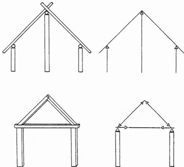
Abb. 48: Schematische Darstellung der Rofen-Pfetten-Bauweise (oben) und der Sparrenbauweise (unten). (Aus Masuch/Ziessow 1983.)
