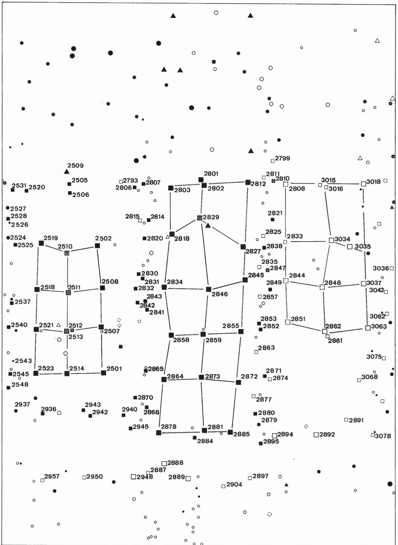
Abb. 35: Latrigen VI-Riedstation. Pfahlplan im Bereich der Häuser 1 und 2 (3393 v.Chr.) sowie Haus 3 (3392 v.Chr.). Die Pfahlnummern entsprechen den Dendro-Nummern/Messkurven auf den Abbildungen 36–38. M. 1:100. Legende der Signaturen siehe S. 45.
