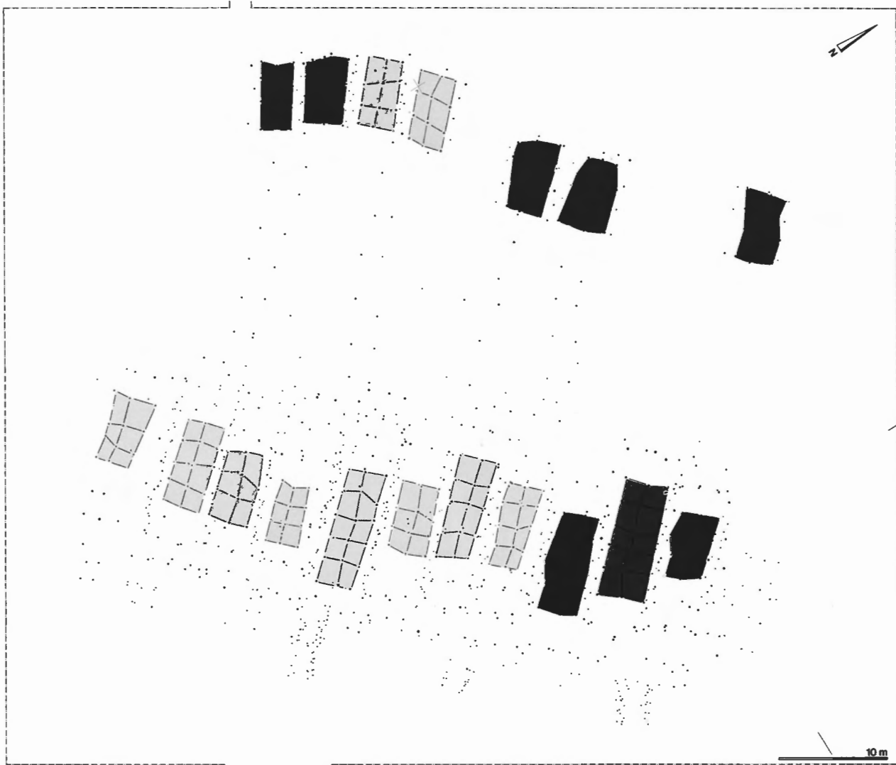
Abb. 32: Lattrigen VI-Riedstation. Baugeschichte. Dunkler Raster: Hausgrundrisse des Schlagjahres 3390 v.Chr.; heller Raster: bereits bestehende Gebäude. M. 1:500.
