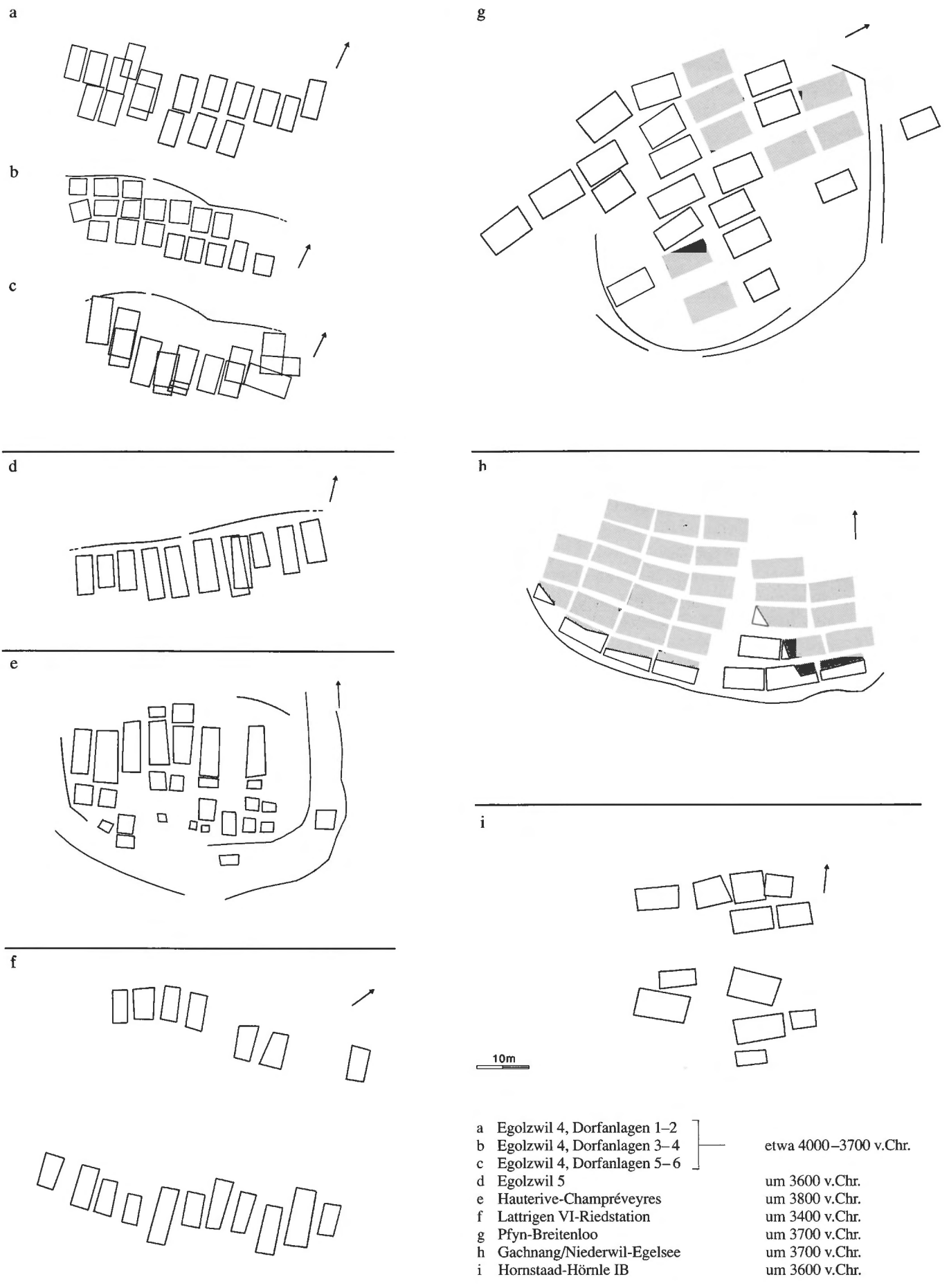
Abb. 54: Dorfgrundrisse der Cortaillod-Kultur (a-f) und der Pfyn Kultur (g-i; Raster = ergänzte Häuser). M. 1:1000.
