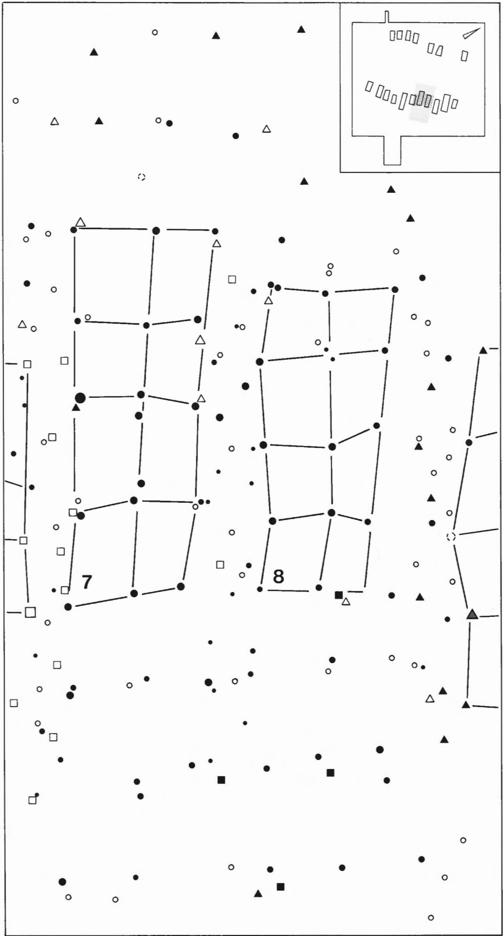
Abb. 40: Lattigen VI-Riedstation. Pfahlplan im Bereich der Häuser 7 und 8 (3391 v.Chr.). M. 1:100. Legende der Signaturen siehe S. 45.
