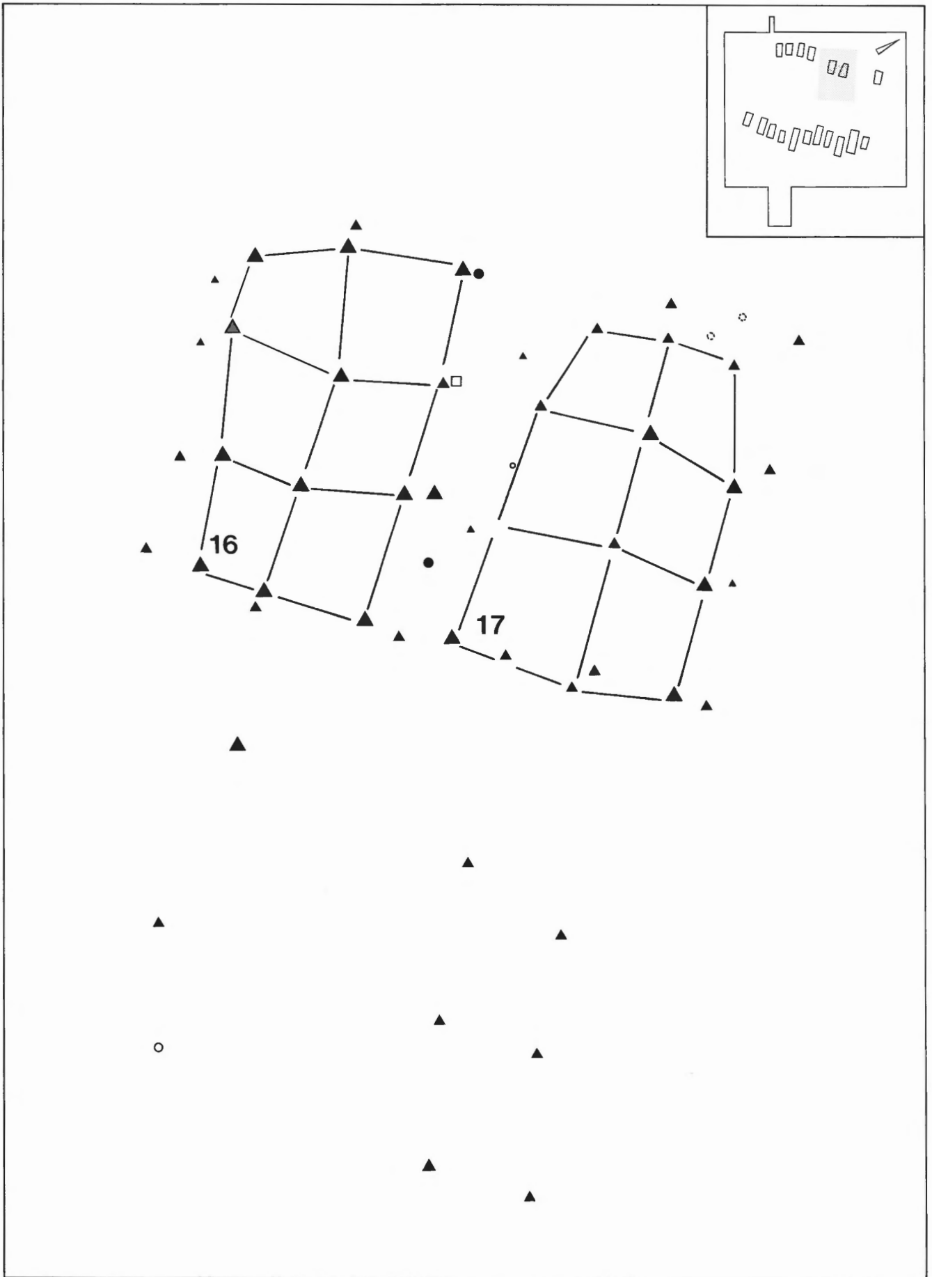
Abb. 44: Lattrigen VI-Riedstation. Pfahlplan im Bereich der Häuser 16 und 17 (3390 v.Chr.). M. 1:100. Legende der Signaturen siehe S. 45.
