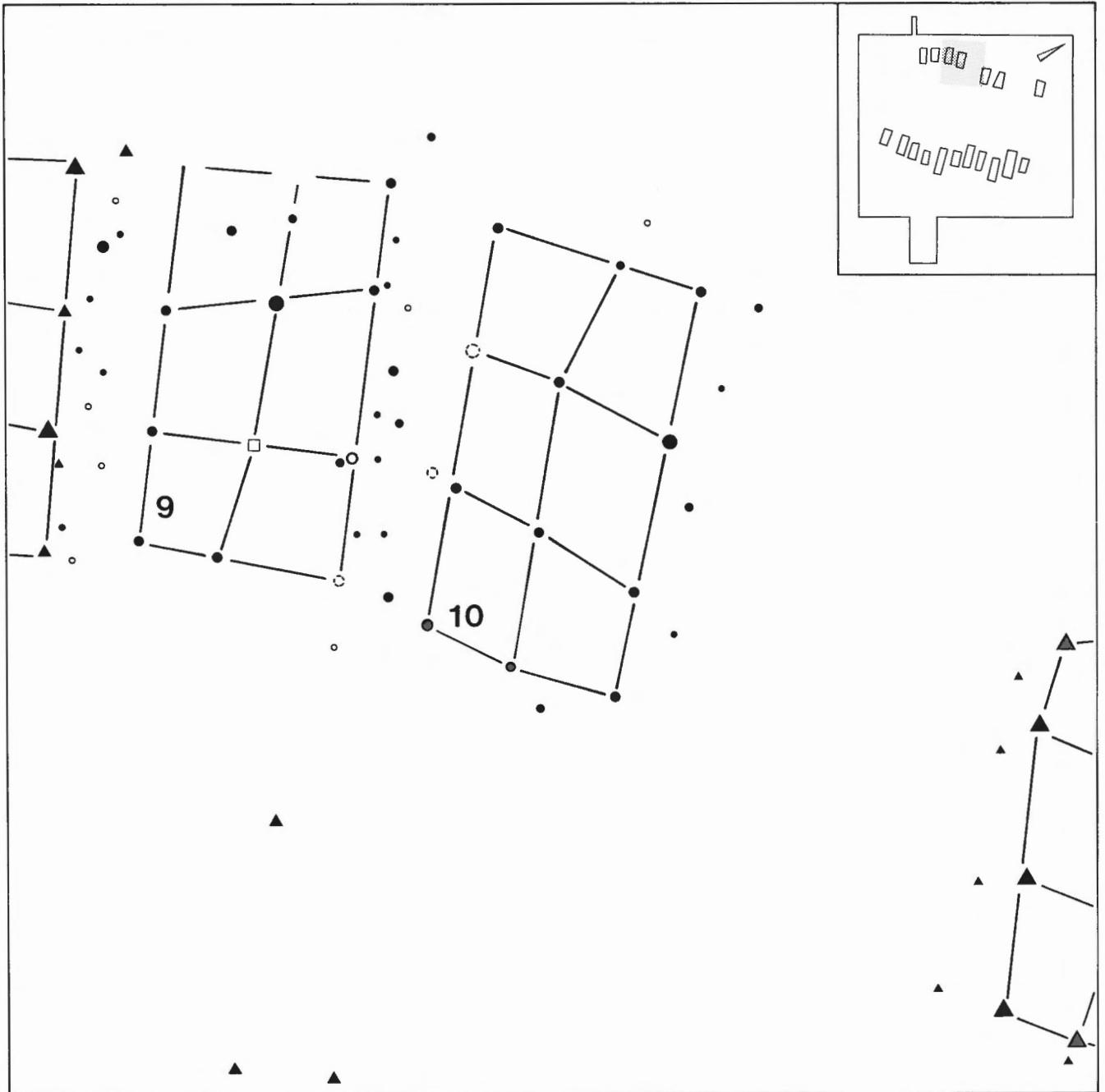
Abb. 41: Lattigen VI-Riedstation. Pfahlplan im Bereich der Häuser 9 und 10 (3391 v.Chr.). M. 1:100. Legende der Signaturen siehe S. 45.
