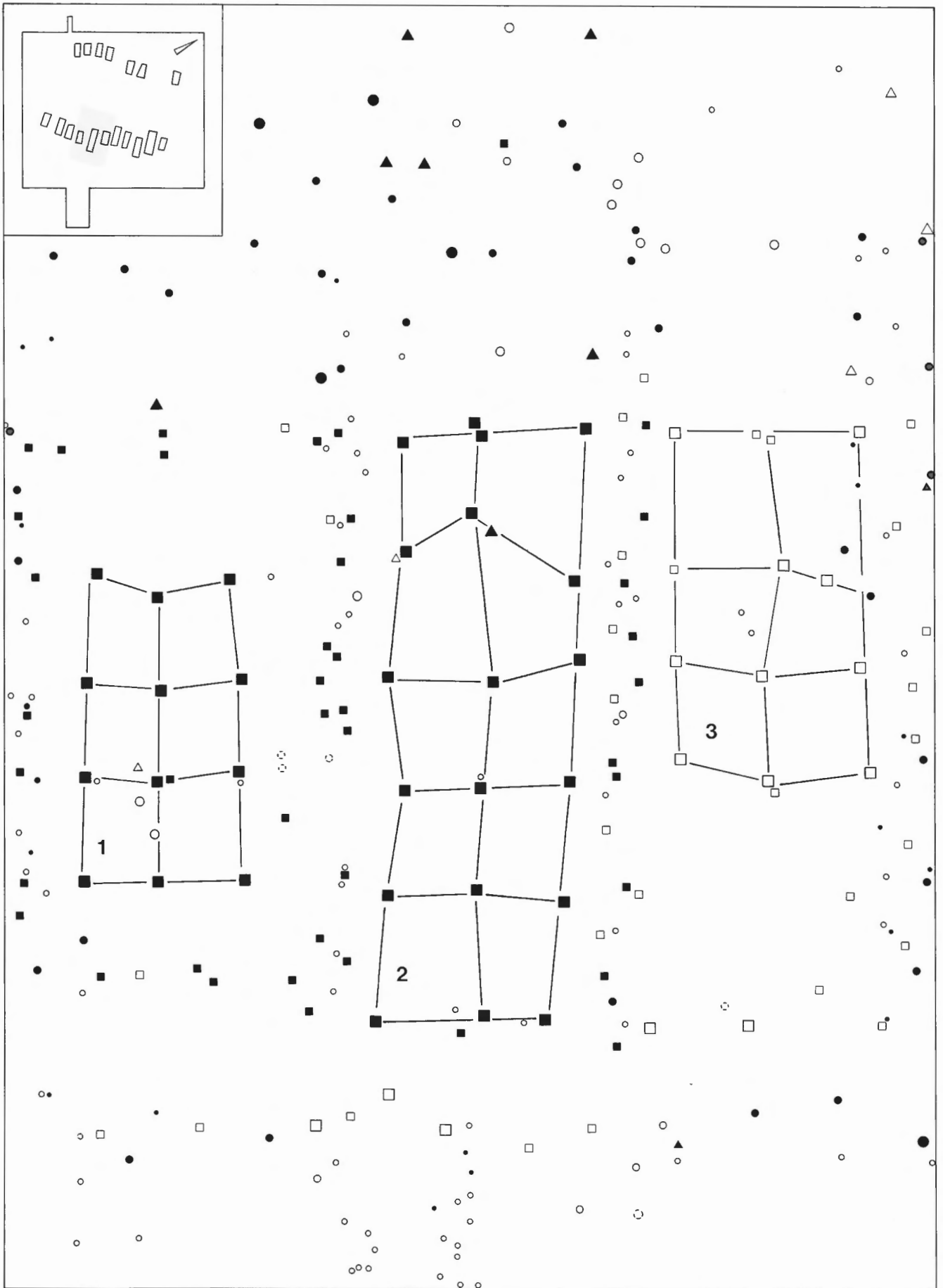
Abb. 34: Lattigen VI-Riedstation. Pfahlplan im Bereich der Häuser 1 und 2 (3393 v.Chr.) sowie Haus 3 (3392 v.Chr.). M. 1:100. Legende der Signaturen siehe S. 45.
