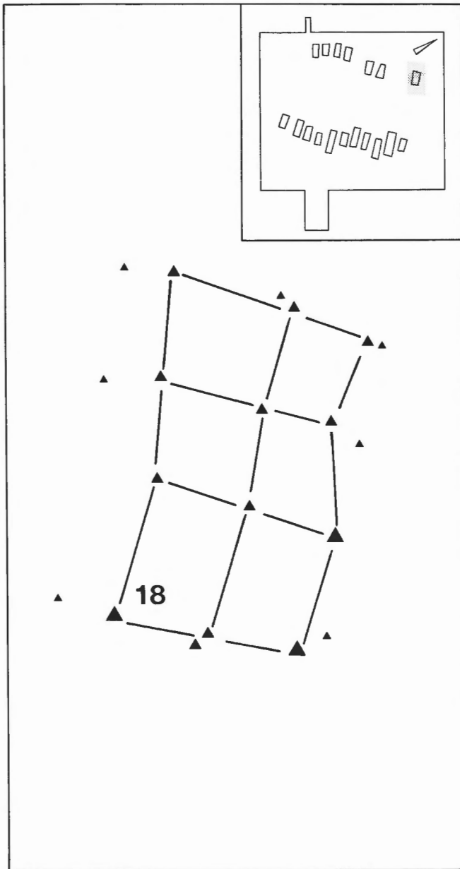
Abb. 45: Latrigen VI-Riedstation. Pfahlplan im Bereich des Hauses 18 (3390 v.Chr.). M. 1:100. Legende der Signaturen siehe unten.
