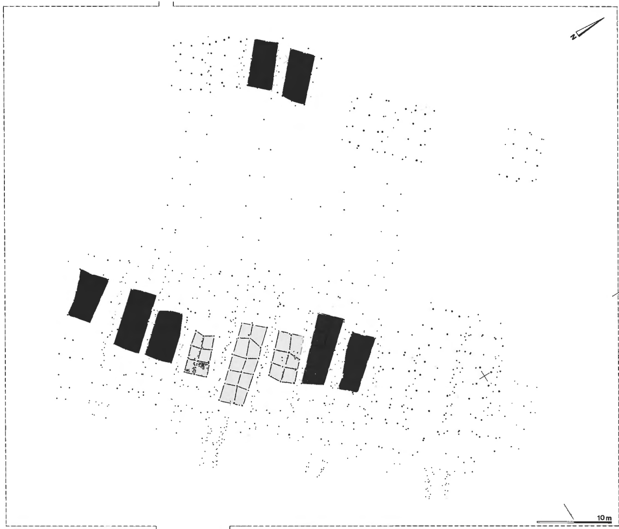
Abb. 31: Lattrigen VI-Riedstation. Baugeschichte. Dunkler Raster: Hausgrundrisse des Schlagjahres 3391 v.Chr.; heller Raster: bereits bestehende Gebäude. M. 1:500.
