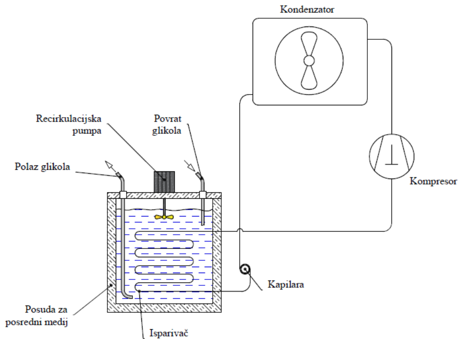
Slika 1.5 Uređaj za hlađenje posrednog medija
