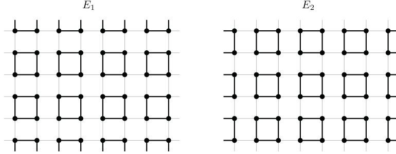
Fig. 9. Spanning subgraphs of T_{8,6} for Lemma 19.
