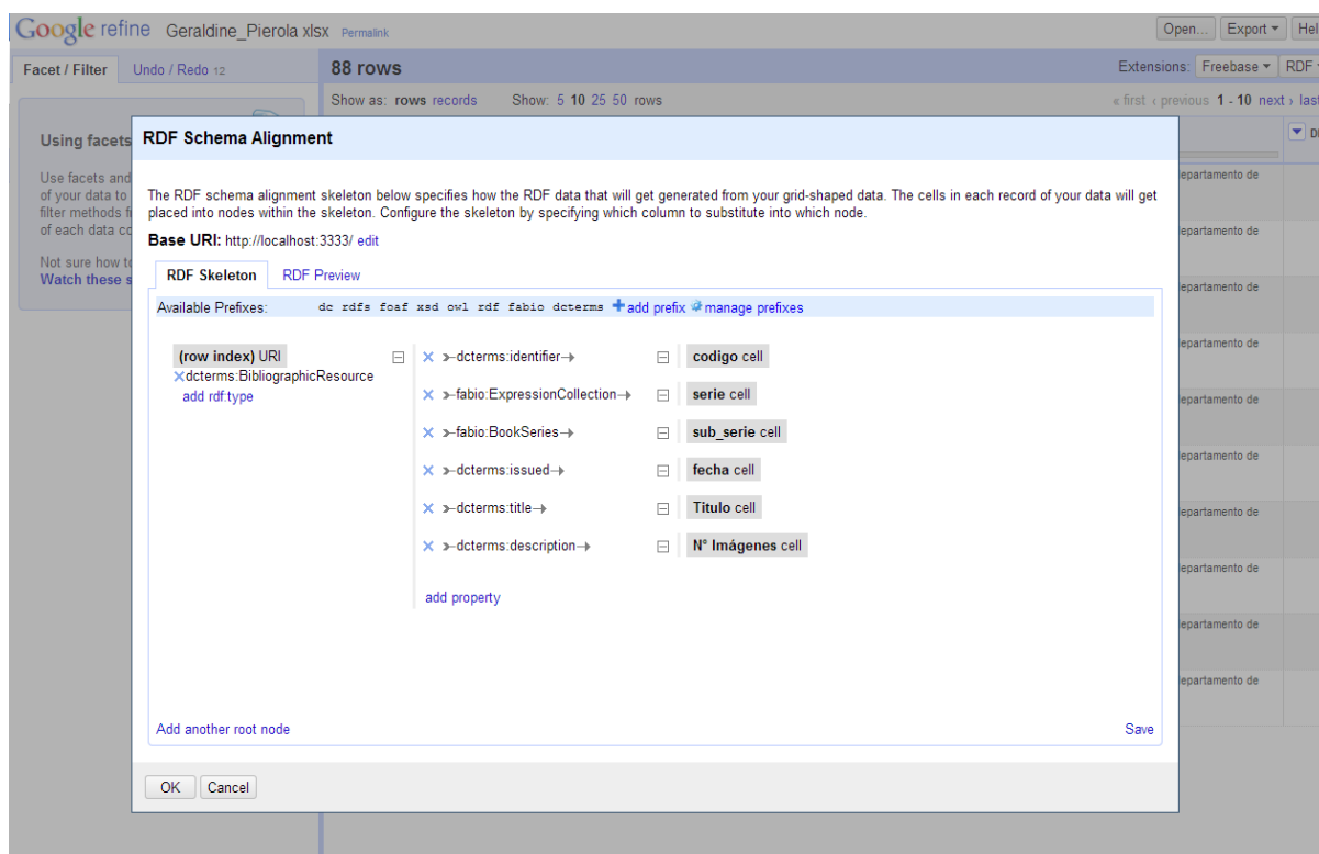
Figura 37. RDF Skeleton de datos, Colección Piérola
