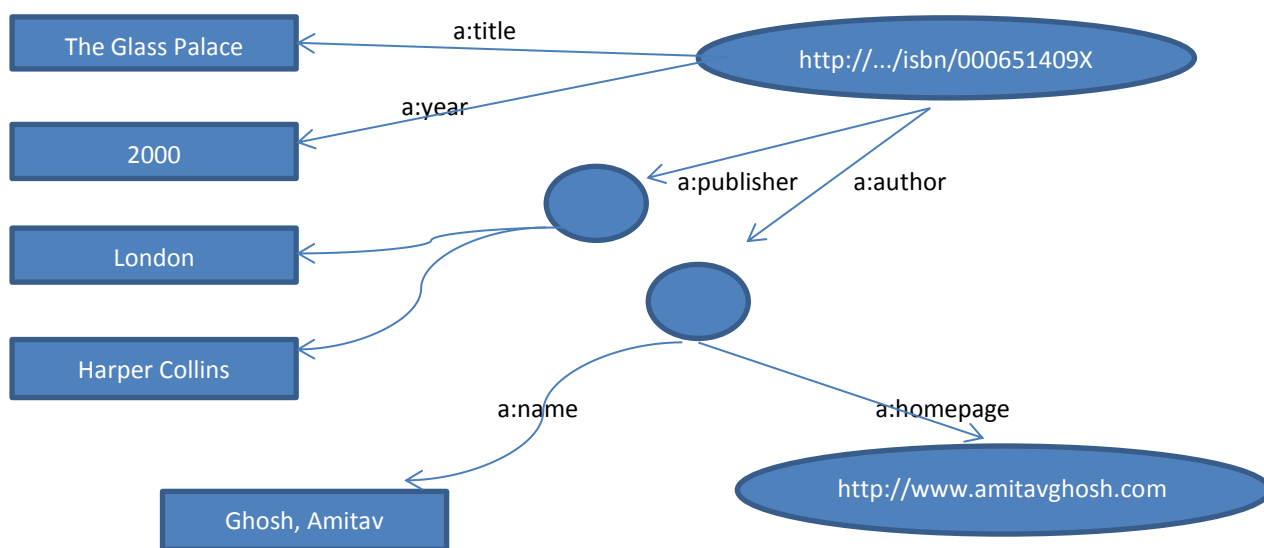
Figura 10. Grafo RDF (Ivan Herman, 2009)
