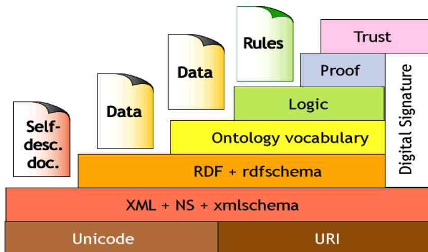
Figura 2. "Capas" de la Web Semántica (W3C)
