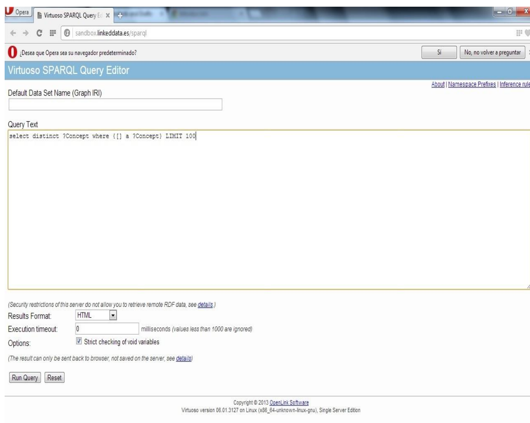
Figura 12. Virtuoso, punto de acceso SPARQL (Corcho y García, 2013) Virtuoso SPARQL Query Editor http://sandbox.linkeddata.es/sparql
