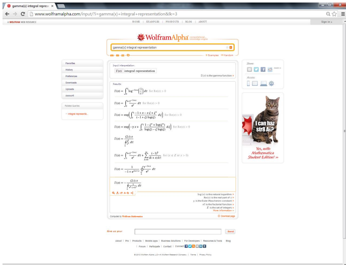
Figura 14. Ejemplo "Representación Integral de Gamma"
