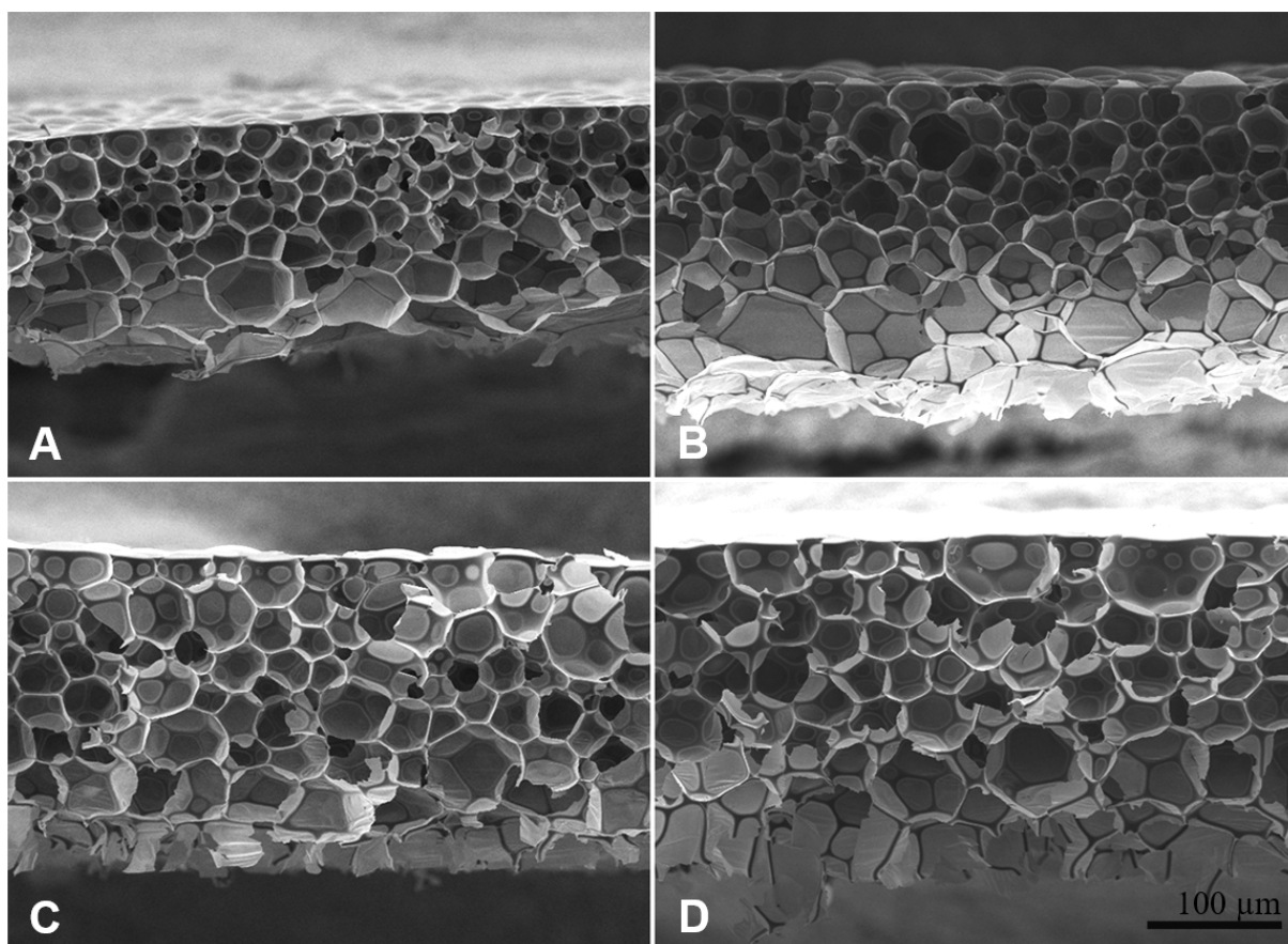
Joonis 12. Skaneeriva elektronmikroskoobi abil saadud kujutised erinevate lahustitega valmistatud vahukilede ristlõigetest, kus A – metanool, B – etanool, C – 1-propanool, D – 1-butanoool.
