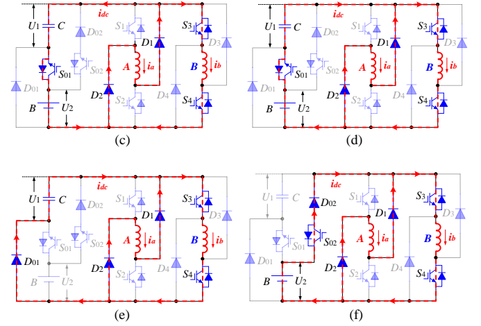
Fig. 7. Demagnetization modes of the proposed converter. (a) Demagnetization mode D1. (b) Demagnetization mode D2. (c) Demagnetization mode D3. (d) Demagnetization mode D4. (e) Demagnetization mode D5. (f) Demagnetization mode D6.
