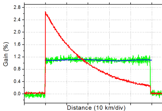
Fig. 10. Trazas de ganancia experimentales adquiridas para ~50 km de fibra con pulsos de 40 ns. La curva roja muestra el resultado obtenido en estas condiciones con un sistema BOTDA tradicional, frente a la curva verde que es el resultado de un BOTDA asistido por Raman de Segundo orden. La curva azul muestra el resultado de la simulación numérica de la evolución de la ganancia.
