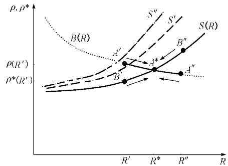
图1 容量-可靠性的相关性分析 Fig. 1 Capacity-reliability correlation analysis
