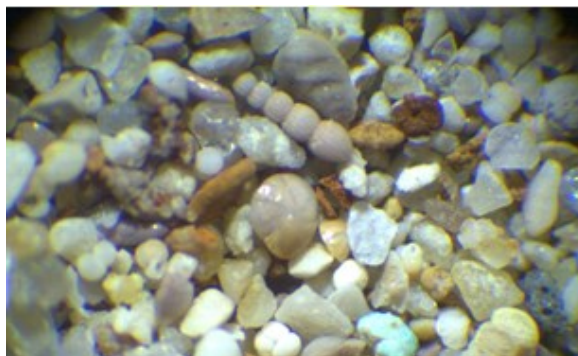
Figura 9. Arriba: fotografía de levigados (izquierda) (fracción 125 micras, materiales de la Cuenca del Bajo Segura); abajo: arenas (playa de Rodas, islas Cies). Imágenes tomadas con la Cámara EOS 500D – microscopio OPTECH modelo B3
