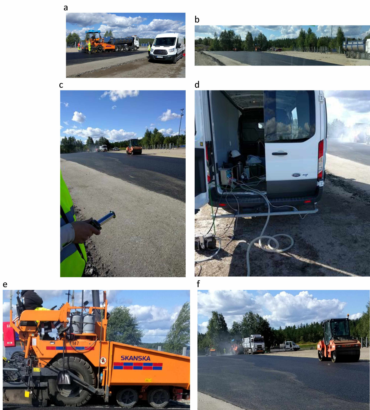
Kuva 3: Valokuvia mittauskohteesta 2.
