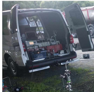
Kuva 2: Valokuvia mittauskohteesta 1. Mittalaitteet oli sijoitettu pakettiautoon (b) ja auto pysäköitiin lähelle asfaltoitavan alueen reunaa.
