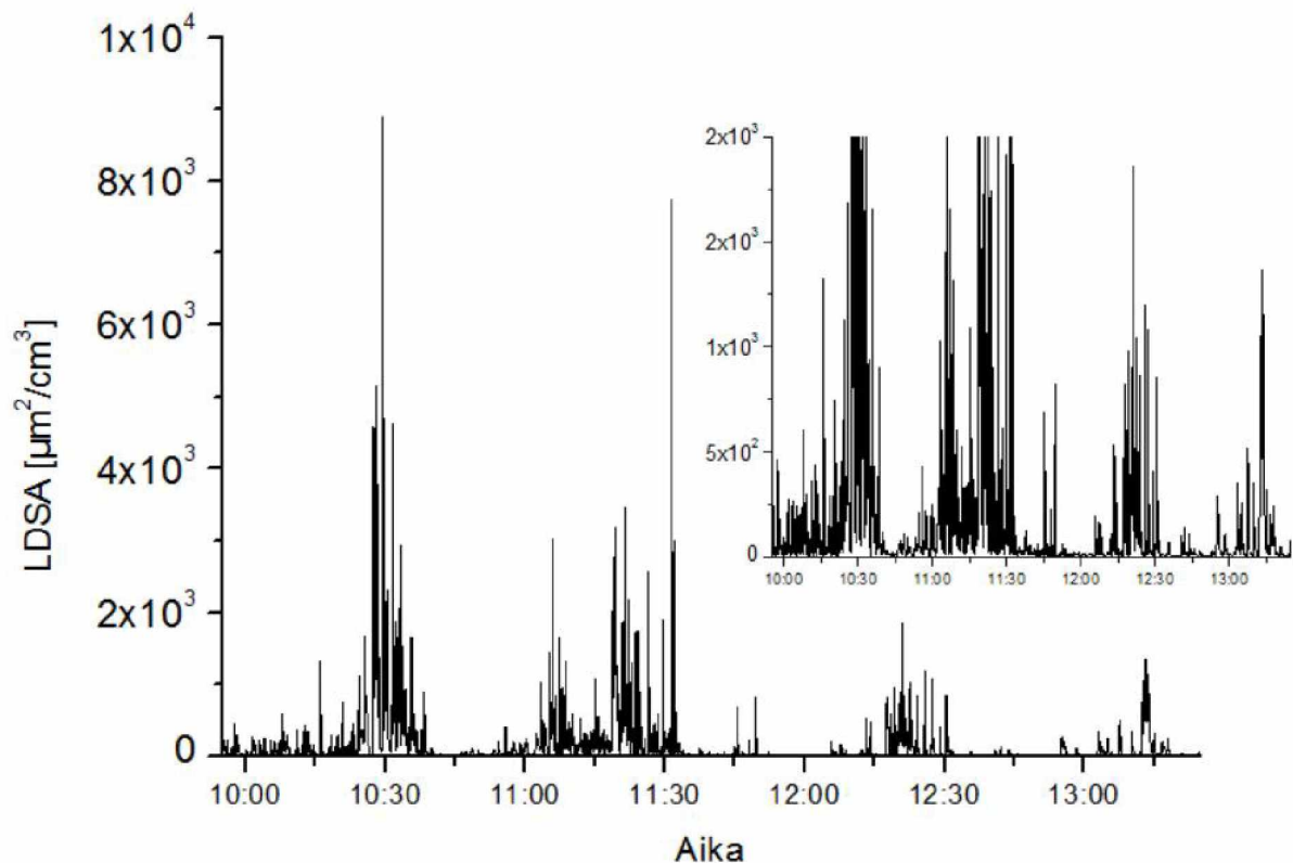
Kuva 17: Aikasarja LDSA-pitoisuudesta (NSAM-alveolar). Sisemmässä kuvassa pienempi y-akseli.
