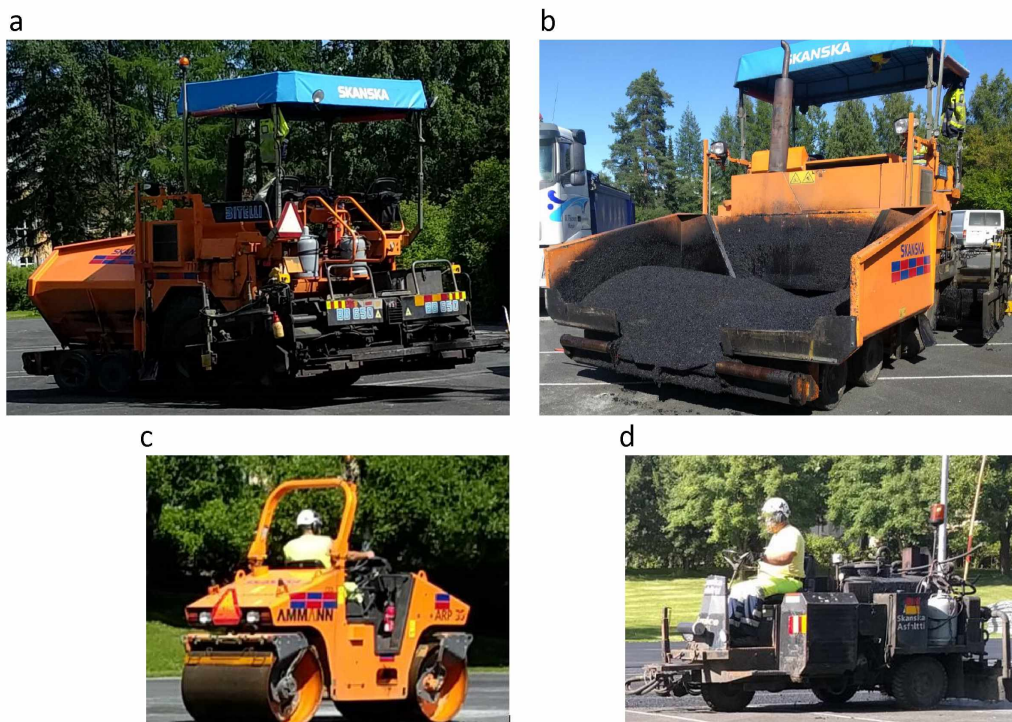
Kuva 1: Valokuvia asfaltointityökoneista (kohde 1). a) ja b) levitinkone, c) jyrä, d) liimamopo.
