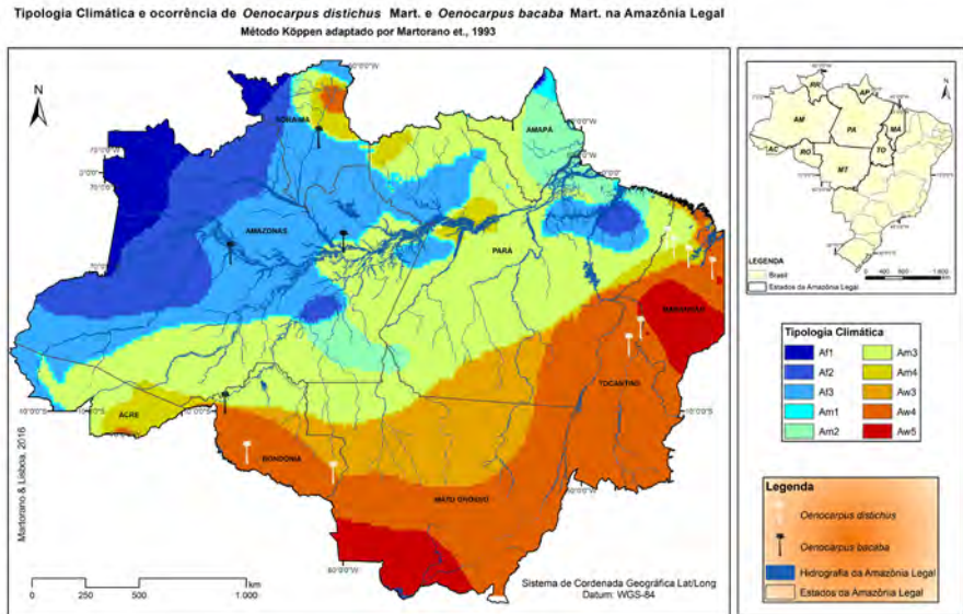
Figura 8. Ocorrência natural associada à tipologia climática na Amazônia Legal.
