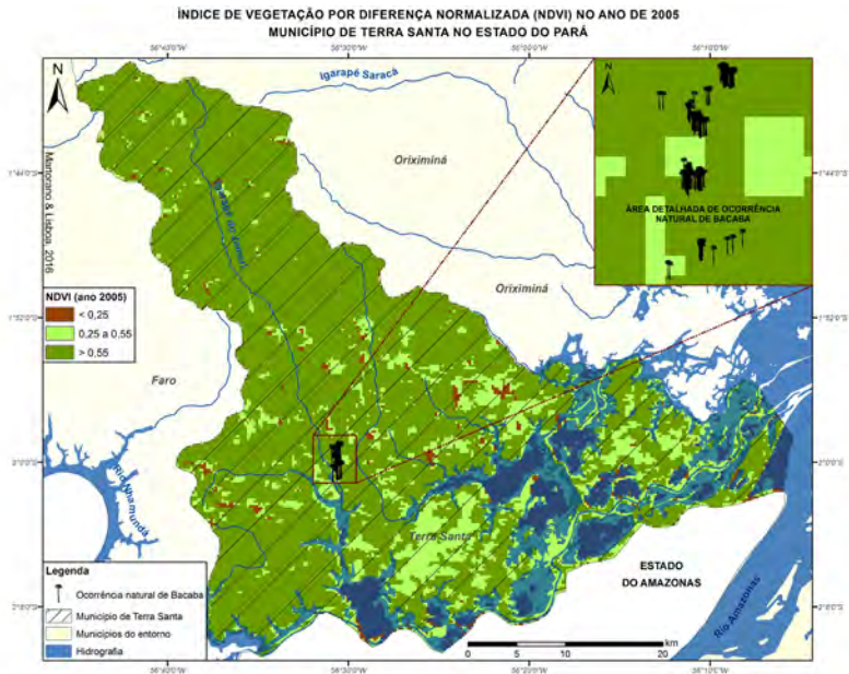
Figura 17. Faixas de NDVI em outubro de 2005, em Terra Santa, Pará.
