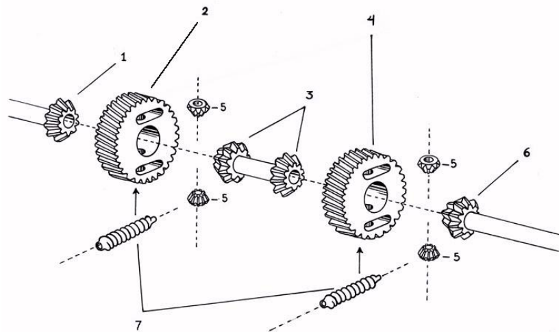
Figura 8. Visão explodida das peças para o modelamento de custo.
